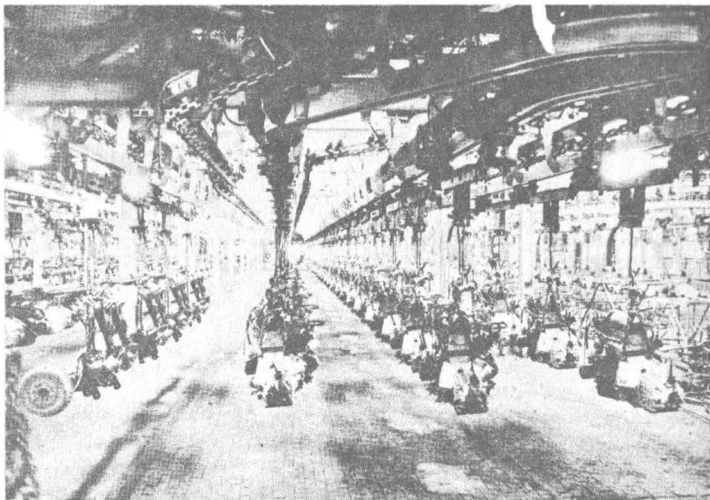
Togliattigrad'daki Fiat tesisleri.
