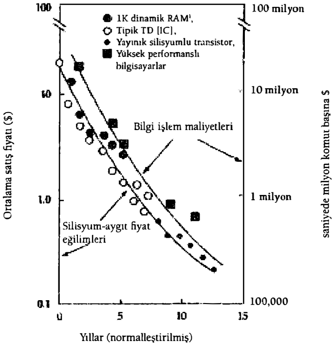
ŞEKİL 9.2. Paralel azalmalar bilgisayarların maliyetinin yarı iletken maliyetlerine nasıl bağlı olduğunu gösteriyor
