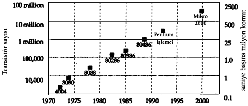
ŞEKİL 9.1. Intel mikro-işleyicilerin evrimi, 1970-2000
