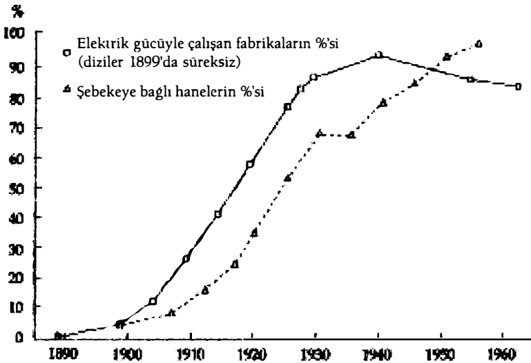
ŞEKİL 7.2. ABD'de elektrifikasyon, 1890-1960
