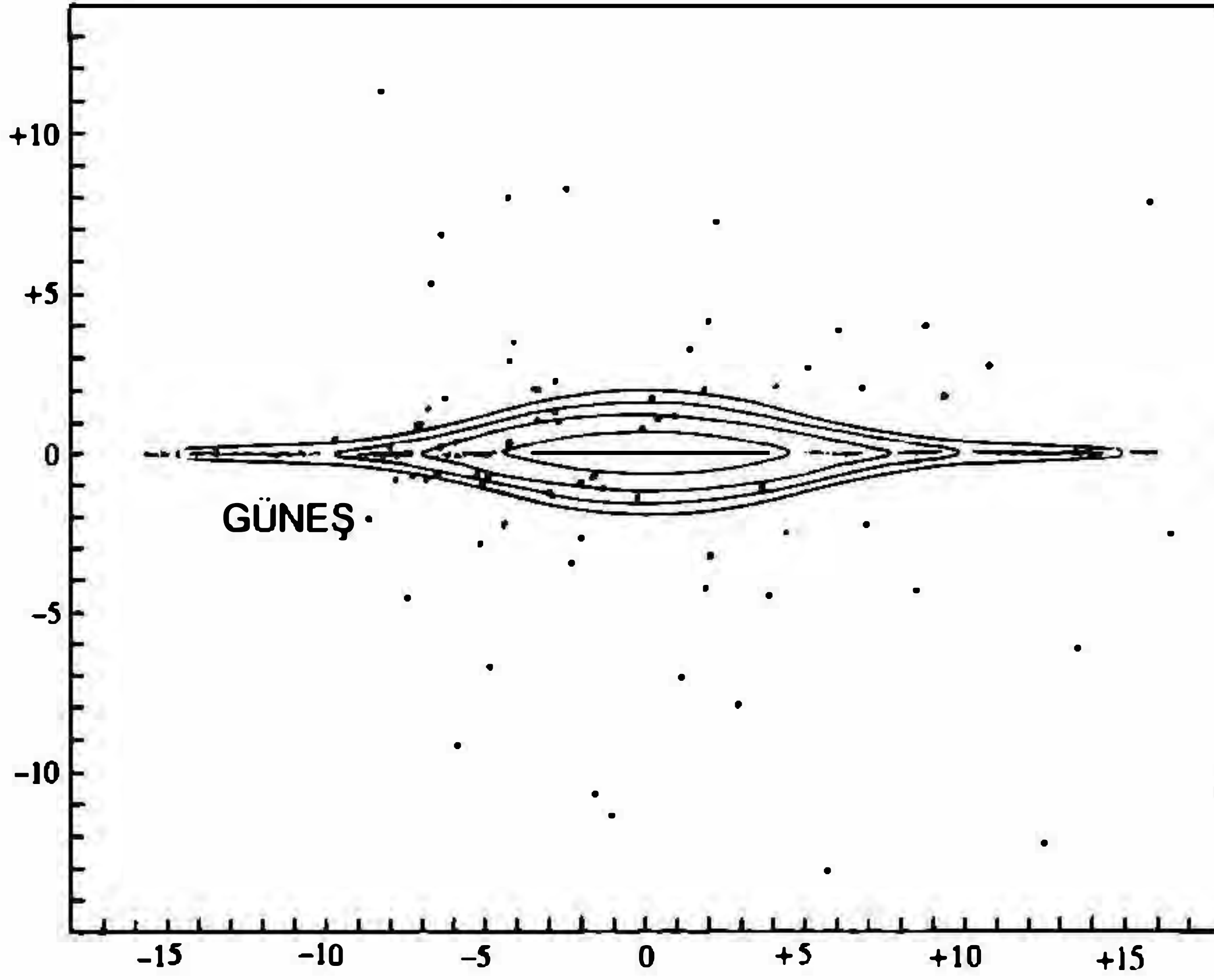
Şekil 7. Samanyolu'ndaki mesafeler ve güneşimizin Samanyolu'ndaki konumu.
