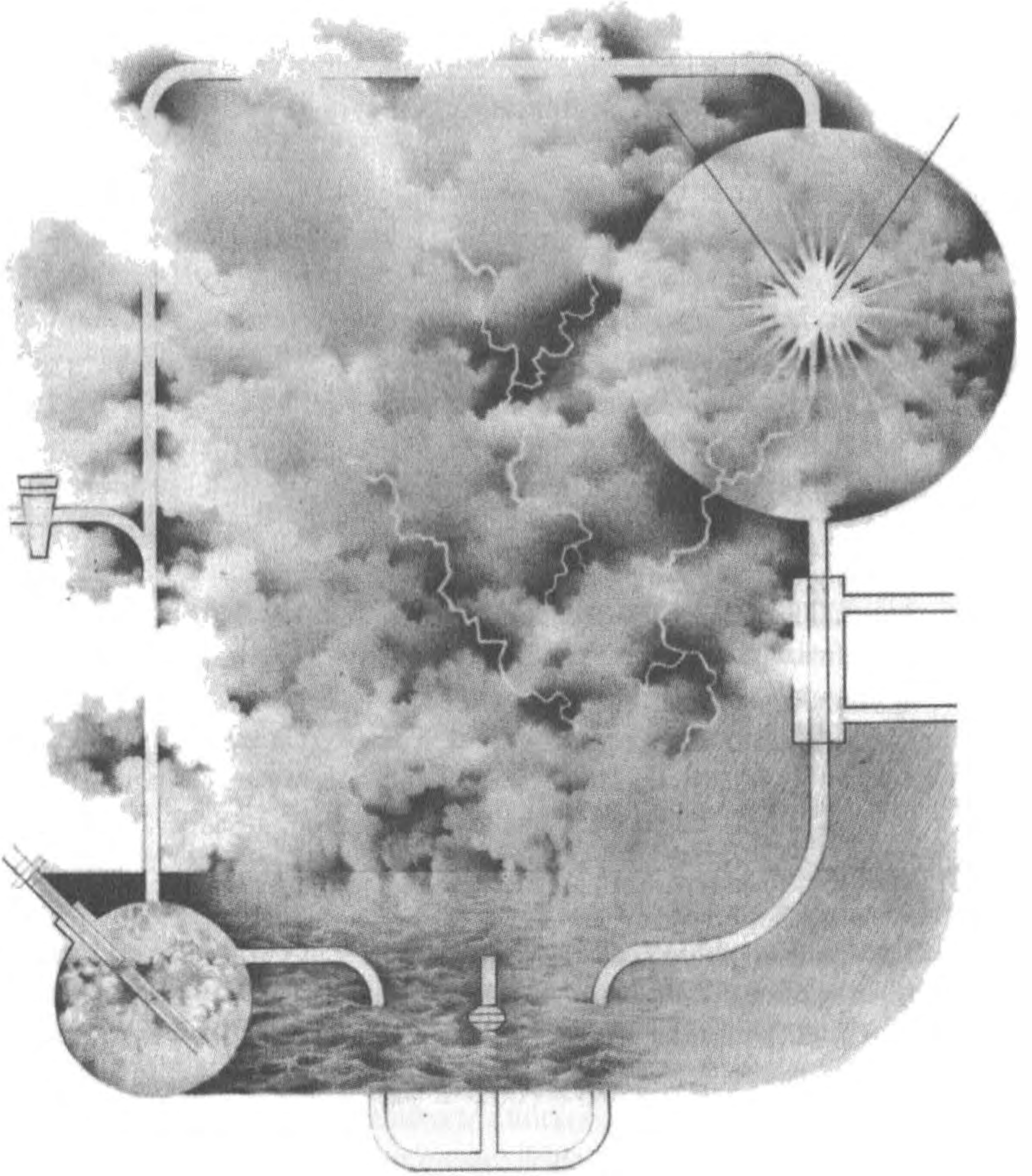
Şekil 11. İlkel atmosferde yaşananları temsil eden Miller deneyi.
