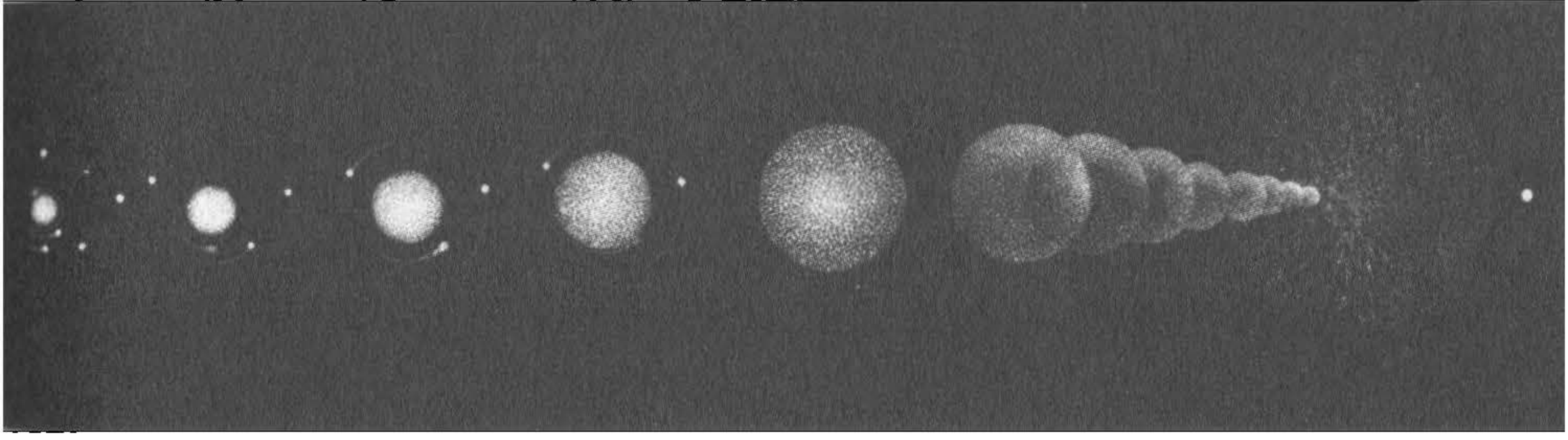
Şekil 8. Bir yıldızın oluşum sürecindeki dönüşüm aşamalarının çizimi.
