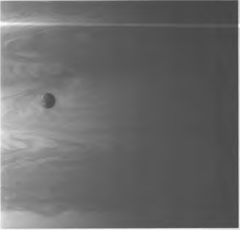
FOTOĞRAF 13 Jupiter'in Uydusu Io, NASA/JPL/CICLOPS
