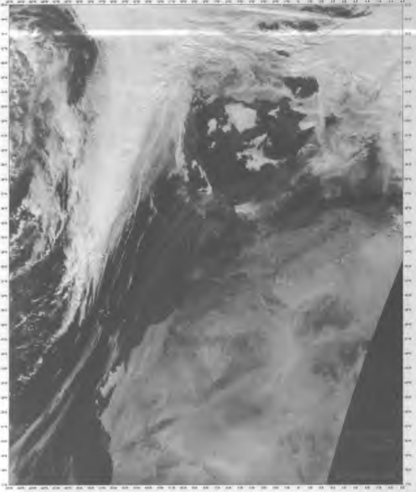
FOTOĞRAF 11 Fas Üzerinde Kum Fırtınası, İspanya, NASA
