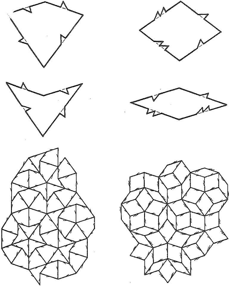
Şekil 4.12. Her biri sadece periyodik-olmayarak kaplayabilen iki çift karo ('Penrose karo-roları'); ve düzlemin her bir çift-karoyla kaplanmış bölgeleri.
