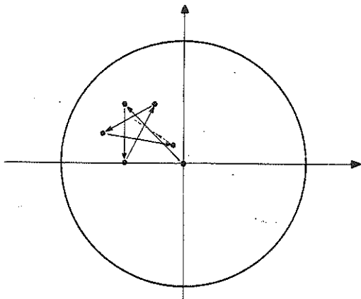
Şekil. 3.12 Eğer Argand düzlemindeki noktalar dizisinin tüm noktaları bir çemberin içine alınabiliyorsa, diziye sınırlı denir. (Şekildeki dizi c = \frac{1}{2} + \frac{1}{2}i 'i sayısından türetilmiştir.
