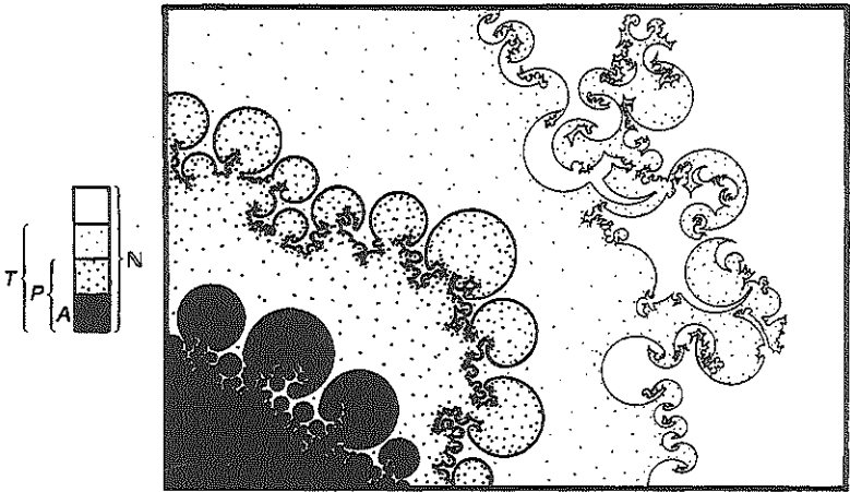
Şekil 4.3. Çeşitli önergeler kümelerinin son derece şematik tasarımı. Sistemde kanıtlanabilir önergeler kümesi P, A gibi, tekrar tekrar sayılabilir olmasına karşın yinelenebilir değildir; doğru önergeler kümesi, T, tekrar tekrar sayılabilir bile değildir.
