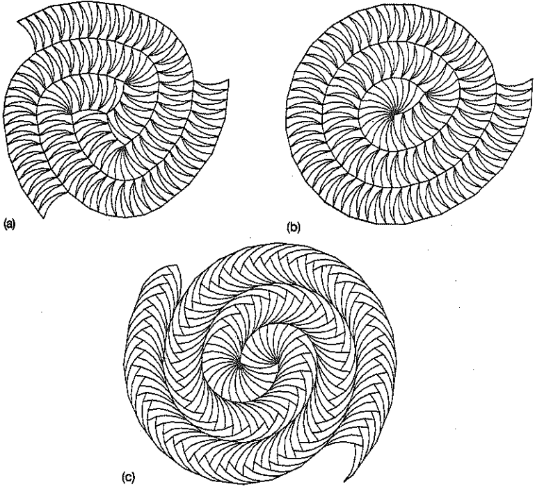
Şekil 4.9. Şekil 4.8'dekinin aynı 'her yöne uzanabilen' biçimi kullanan üç ayrı periyodik olmayan 'helisel' karo kaplama.
