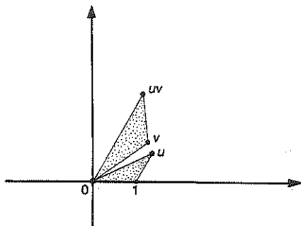
Şekil 3.11: u ve v kompleks sayılarının çarpımı uv , 0 , v , uv tarafından oluşturulan üçgenin, 0 , 1 , u tarafından oluşturulan üçgene benzerliğini sağlar. Buna özdeş olarak, uv 'in 0 'dan uzaklığı, u ve v 'in 0 'dan uzaklıklarının çarpımına eşittir; 0 , 1 , uv uv 'in reel eksen (yatay eksen) ile yaptığı açı, u ve v noktalarının bu eksenle yaptıkları açıların toplamıdır.
