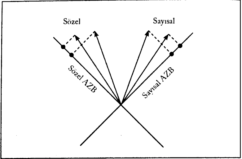
Şekil 4: Birincil ve ikincil basit yapı eksenleri, g ortadan kaybolmuş, AZB: asal zihinsel beceriler için kısaltma
