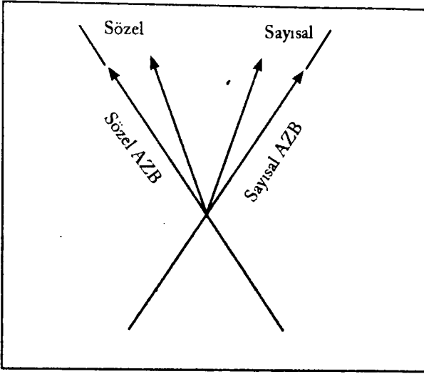
Şekil 5: Birincil ve ikincil eğik basit yapı eksenleri, AZB: asal zihinsel beceriler için kısaltma
