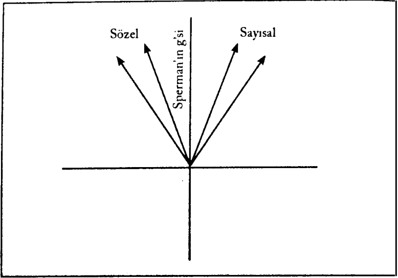
Şekil 3: Birinci ve ikinci eksenler, asal bileşenin yönelimi
