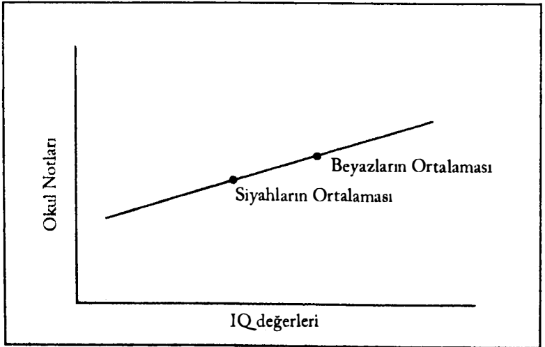
Şekil 2: İstatistiksel yansız bir test.
