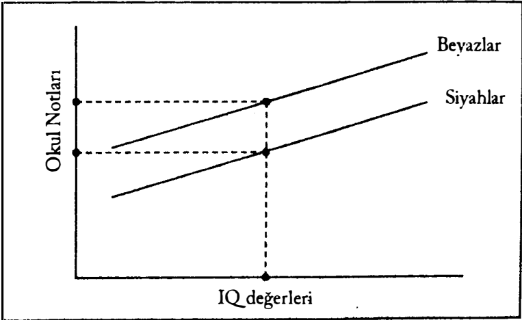
Şekil 1: İstatistiksel olarak yanlı bir test. Aynı IQ değeri siyahlar ve beyazlar için farklı notlara işaret ediyor.
