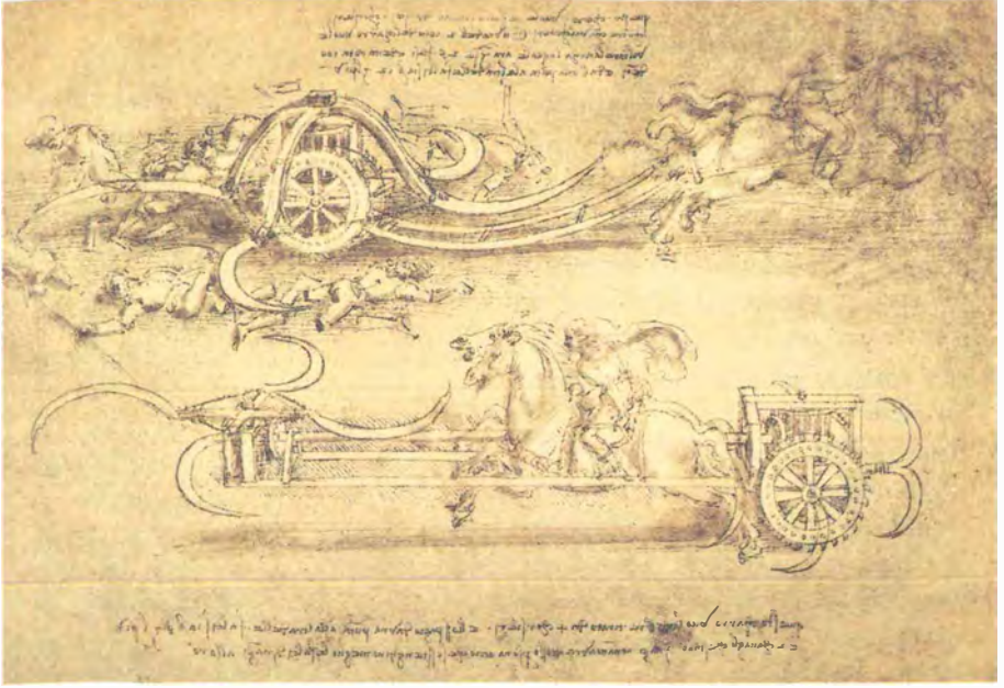
Leonardo da Vinci, Tırpanlı araba çizimi , 1487-1490, Torino, Biblioteca Reale
