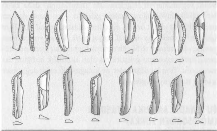
Şekil 5.3 Geometrik Kebaran mikrolitleri. Kebaranlar ok ucu olarak kullandıkları bu parçaları büyük miktarlarda ürettiyordu.
