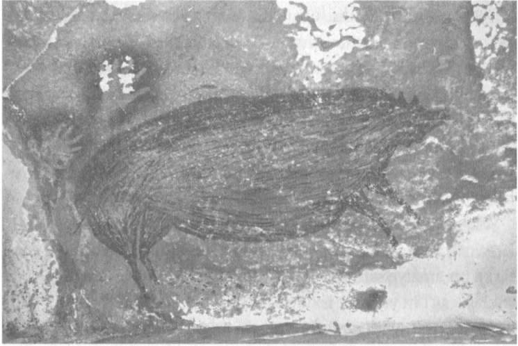
Şekil 3.4 Leand Tedongnge Mağarası'nda bulunan, el izleriyle beraber görülen siğil domuzu resmi, Sulawesi, Endonezya, y. 45.500 yaşında. Maxime Aubert'in izniyle kullanılmıştır.
