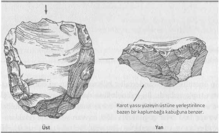
Şekil 2.6 İnce ve çok keskin bir yonga üreten, özenle hazırlanmış bir "Levallois" karotu.
