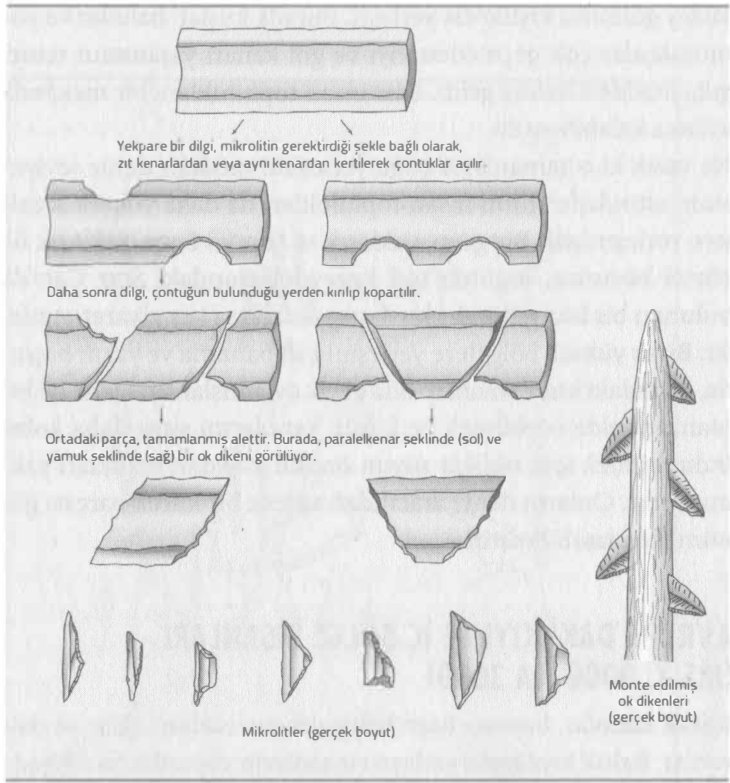
Şekil 5.2 Mikrolitler. Bir mikrolit üretiminin evreleri. Bir dilgide çontuk açılması ve alet biçimlenince ana parçanın koparılmasıyla üretilen, küçük bir ok dikenini veya benzeri bir alet.
