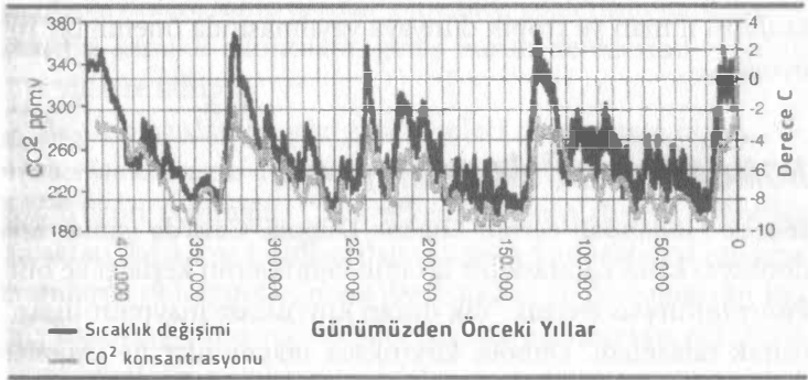
Şekil 2.1 Buzul Çağı iklim değişikliği. Antarktika'daki Vostok buz karotunun ortaya çıkardığı, son 420 bin yıl içerisinde gerçekleşmiş iklim dalgalanmaları, hem sıcaklığı hem de CO 2 değişimlerini göstermektedir.
