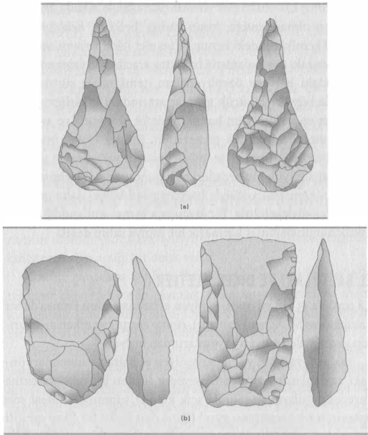
Şekil 2.3 El baltası teknolojisi. (a) Swanscombe, İngiltere'den Aşölyen el baltası (gerçek boyutunun üçte biri) (b) Angola ve Zambiya'dan iki Aşölyen satır (ikisi de gerçek boyutunun yarısı). Satırların et kesme aletleri olarak kullanıldığı düşünülüyor. Modern deneylerde kaba, yekpare kenarlarının hayvanın derisini yüzme ve parçalara ayırmakta etkili olduğu anlaşıldı.
