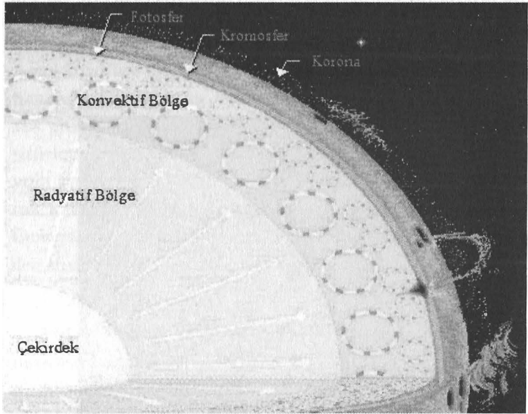
Güneş'in bugünkü iç yapısı.
