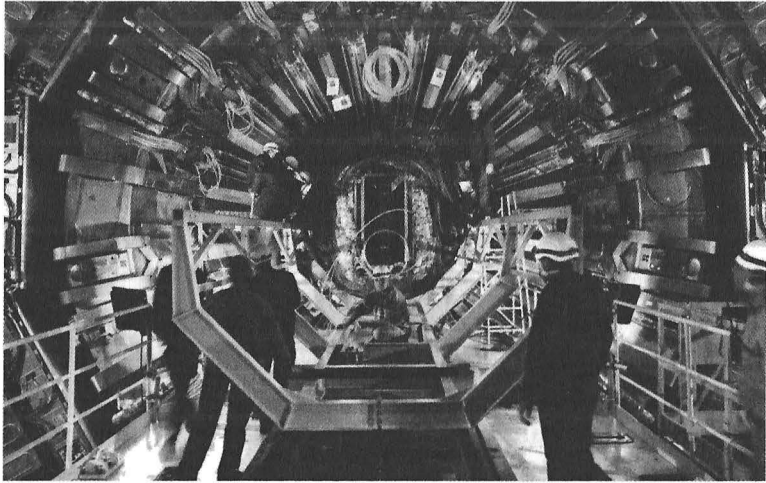
Hadron Çarpıştırıcısı/Cern
