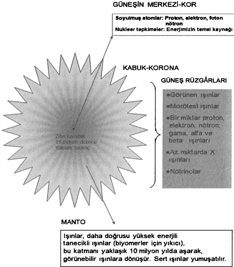
Güneşin bugünkü iç yapısı.
