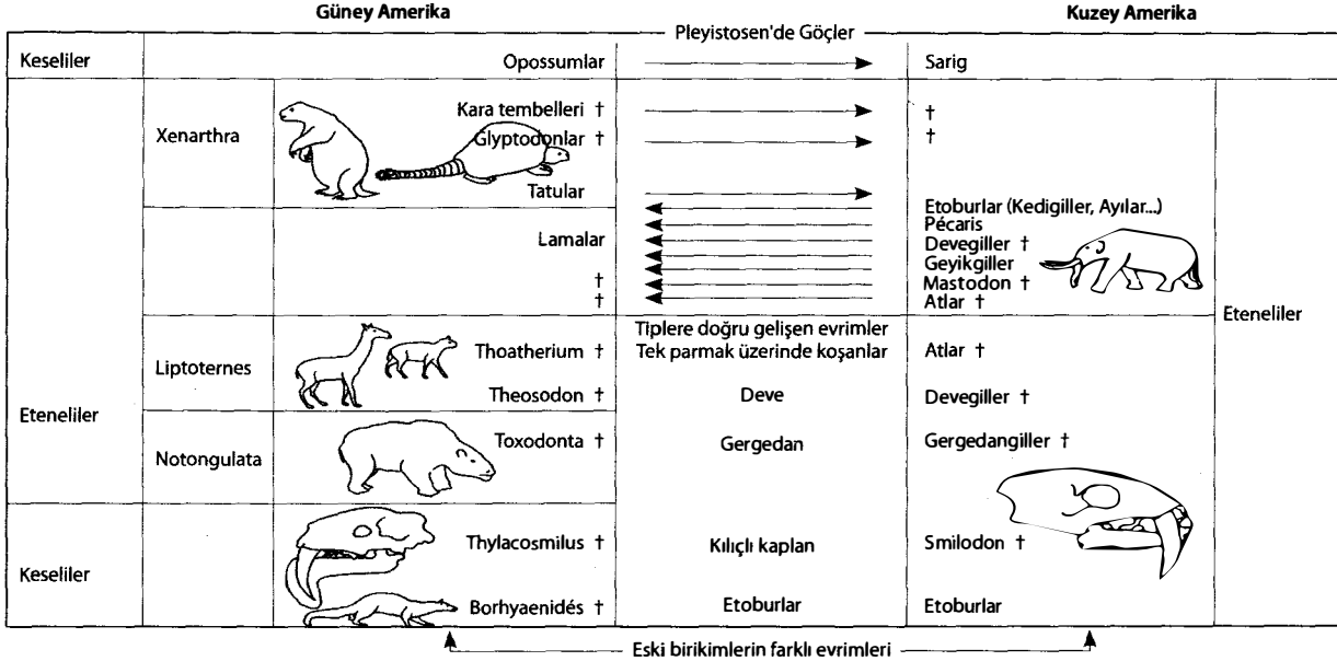
Şekil 11. Güney Amerika Memliler Tarihi Üzerine Olgular. Plio-Pleistosen'de iki Amerika arasındaki bağlantı Orta Amerika yer kabuğunun kabarmasıyla yeniden oluşmuştur. Bunun sonucunda da bazı türler ayıklanmış, bazıları yaşamlarını sürdürmüştür.
