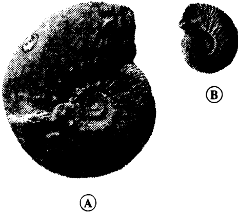
Şekil 20. Ammonitlerde cinsel çiftbiçimlilik: kosmoceras baylei (A) ve guliemiceras gulielmii (B). Bunlar iki farklı cins olarak tanımlanmıştır, günümüzde ise daha çok aynı türün iki cinsiyetine denk düştükleri kabul edilir. Büyük boyutlu biçim (macroconque) dişi, küçük boyutlu biçim (microconque) erildir (Tintant’dan alınmıştır).
