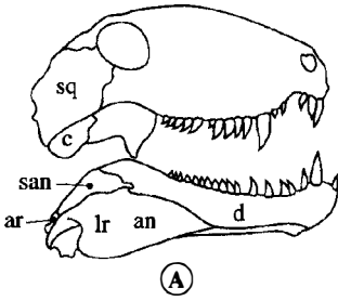
Şekil 47. A- Permiyen dimetrodon 'u pelycosauria'nın (memeli sürüngen) kafatası; B- Kedinin kafatası; ar, Eklemli; an, köşeli ve parlak yüzeyi (lr); bt, orta kulağı kaplayan timpan kabarcığı; c, Kare; d, Dişler; san, Üst-Köşeli; sq, Skuamosal (A, Romer'den alınmıştır).
