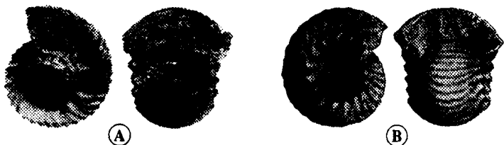
Şekil 41. Kökenleri ve çağları farklı iki ammonit arasındaki morfolojik birlik: A- Erymnoceras (Orta Kalovyen); B- Fagesia (Üst Tebeşir Devri) [Tintant'dan alınmıştır].
