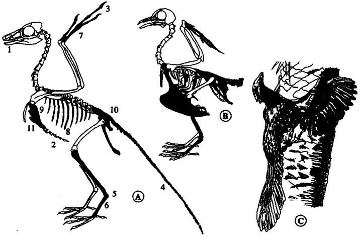
Şekil 30. A- Archaeopteryx iskeleti; B- Günümüzde yaşayan bir kuşun iskeleti, C- Yeni tasarlanmış bir Archaeopteryx (Wellnhofer). Kuramsal olarak Archaeopteryx 'in yapısından günümüzde yaşayan bir kuşun yapısına geçme olanağı sağlayan iskeletlerle ilgili bazı değişiklikler (siyah):
