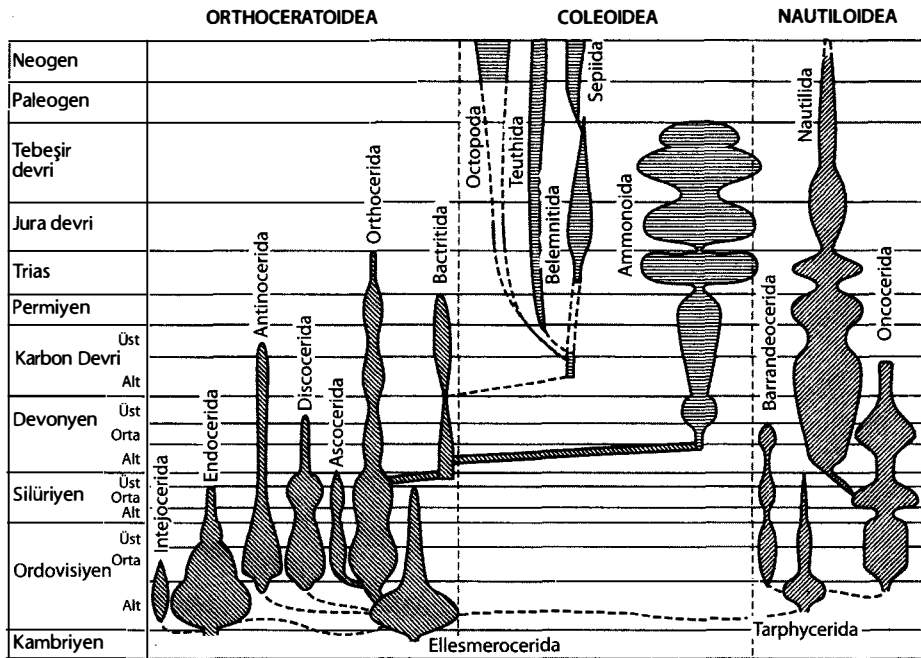
Şekil 44. Kafadanbacaklıların evriminin genel şeması (Tintant'dan alınmıştır).
