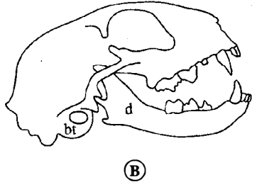
Şekil 47. A- Permiyen dimetrodon 'u pelycosauria'nın (memeli sürüngen) kafatası; B- Kedinin kafatası; ar, Eklemli; an, köşeli ve parlak yüzeyi (lr); bt, orta kulağı kaplayan timpan kabarcığı; c, Kare; d, Dişler; san, Üst-Köşeli; sq, Skuamosal (A, Romer'den alınmıştır).
