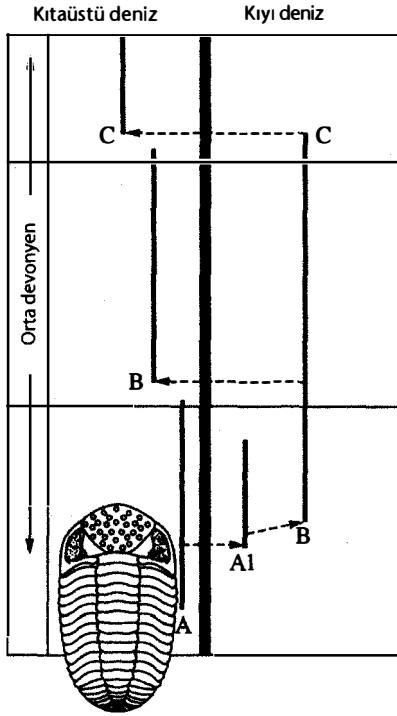
Şekil 24. Devoniyen’de New York eyaletinde trilobit fakops bağlamında gerçekleştirilen gözlemlerden hareketle oluşturulan kesintili dengeler modeli ilkesinin şeması. Kıtaüstü denizde istikrarlı bir A türü marjinal bir denize doğru bir A1 uzantısı gönderir; A1 hızlı bir anagenezden sonra yeni bir B türü olur; bu tür istikrar kazanır ve bölgesini genişleterek A’nın yerini alır (değiştirilmiş biçimiyle Eldredge’den alınmıştır).
