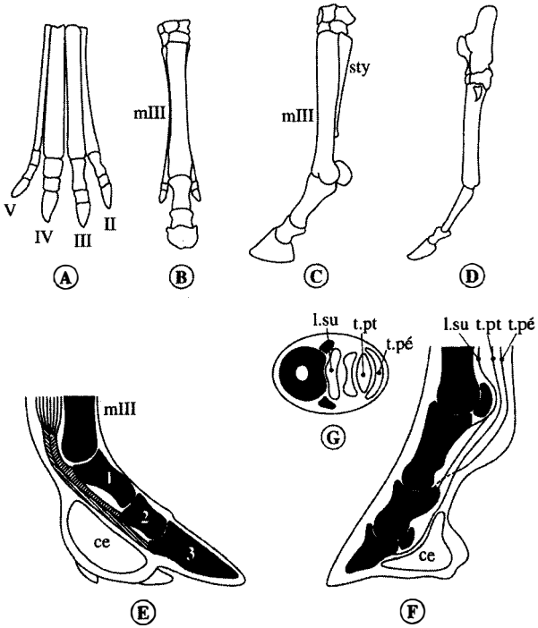
Şekil 46. At ayağının evrimi: A- Hyracotherium 'un 4 aralıklı ön ayağı; merychippus 'un üçparmaklı ayağı; C- bugünkü atların tekparmaklı ayağı; II ve IV aralıkları sivrilmiştir; D- Thootherium 'un tekparmaklı ayağı. Üçüncü Zaman Güney Amerika liptotern'i: II ve IV aralıkları kalmıştır (resimler ölçülü değildir). E- Hyracotherium 'un (E) ve equus 'un (F) ön ayağında esnetici sistemlerin yeniden tasarlanması. Birincisinde parmağı hareket ettiren kaslar, parmak kemikleri hizasına kadar inerler ve bu bölgede kısa tendonlar aracılığıyla hareket ederler; esnek yastık(ce) çok gelişmiştir. İkincisinde kaslar radyus hizasında kalırlar ve parmak kemiklerini iki güçlü tendon (t.pt ve t.pé) aracılığıyla hareket ettirirler; l.su eklemine askıda tutan bağı esnetici sisteme katılır. (G) enine kesiti (xy'ye göre) bu üç yapının olağanüstü gelişimini gösterir: New York American Museum örneklerine göre A, B; Simpson içinde Matthew'den alınan D; değiştirilmiş biçimiyle Camp ve Smith'ten alınan E; F, G yazarlara aittir).
