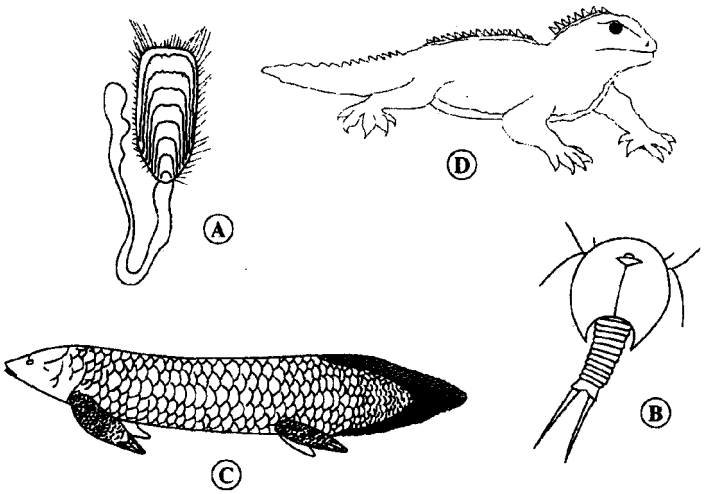
Şekil 26. Bazı "canlı fosiller": A- Lingula , günümüzde Pasifik'te yaşayan kolsuayaklı; B- Triops , tatlı su kabuklu deniz hayvanı; C- Neoceratodus , Avustralya tatlı sulannda yaşayan solungaçlı ve akciğerli "balık"; D- Sphenodon , "sürüngen", Yeni Zelanda Rhyncocephalus 'u.
