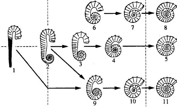
Şekil 3. Evrimsel tersinirlik. Ancyloceras türünden hareketle Aşağı Tebeşir Devri'nin üç ammonit soyu içinde kavkının yeniden yuvarlaklaşması eğilimleri (Wiedmann).
