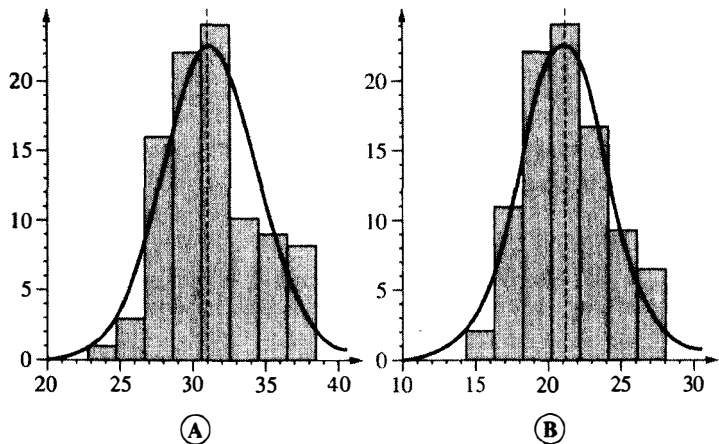
Şekil 13. Melezleşen bir topluluk içinde değişkenliğin dağılımı: Ammonitte ( kepplerites gowerianus ) göbek çapının değişimi (A) ve iç kaburga kemiklerinin sayısının değişimi (B). (Tintant'dan alınmıştır).
