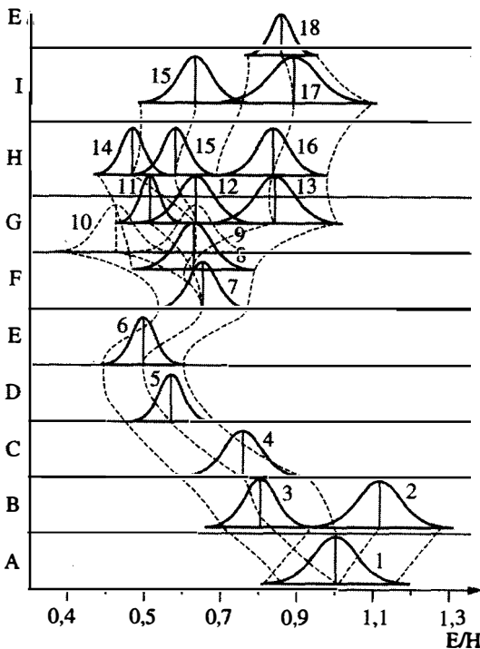
Şekil 18. Ammonit kosmoceras türünde kesitin biçiminin evrimi (Orta Jura Dönemi, 155 milyon yıl). Absislerde yükseklik/genişlik ( E/H ) ilişkisiyle açıklanan kesitin biçimi; ordinatlarda orta (A-G) ve yukarı (H-I) Kalovyen'in sürekli bölgeleri. Jason bölgesinde (B-E) evrim anageniktir ve her "transiant" bir tür olarak düşünülebilir. Coronatum bölgesinde (F-G) soy, farklı topluluklara ayrılır. İlk başta birçok farklı tür doğuran kladogenezler olarak düşünülen bu süreç, bugün çevre değişimelerindeki artışa bağlı özel ve önemli çokbiçimliliğin ortaya çıkışı şeklinde yorumlanmaktadır. Üst Kalovyen'de (H-I) değişkenlik azalır ve soyu çok az değişen tek bir türe indirger (Tintant ve d.).
