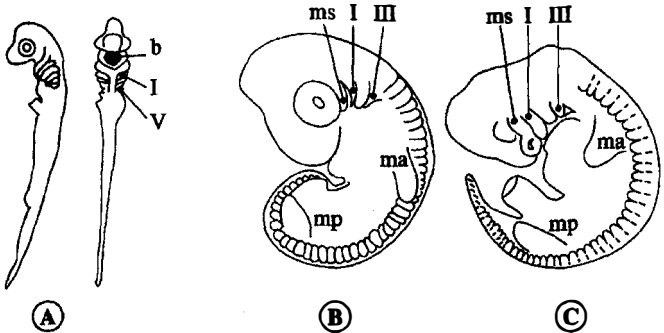
Şekil 4. Embriyolar A-Köpekbalığı; B-Kertenkele; C-Domuz; b, ağız; ön ve arka üyelerin taslakları öü-aü; üç, üst çene taslağı; i-v, içorgan kanalları (A ve B Normentafeln; C, Rugh, basitleştirilmiştir).
