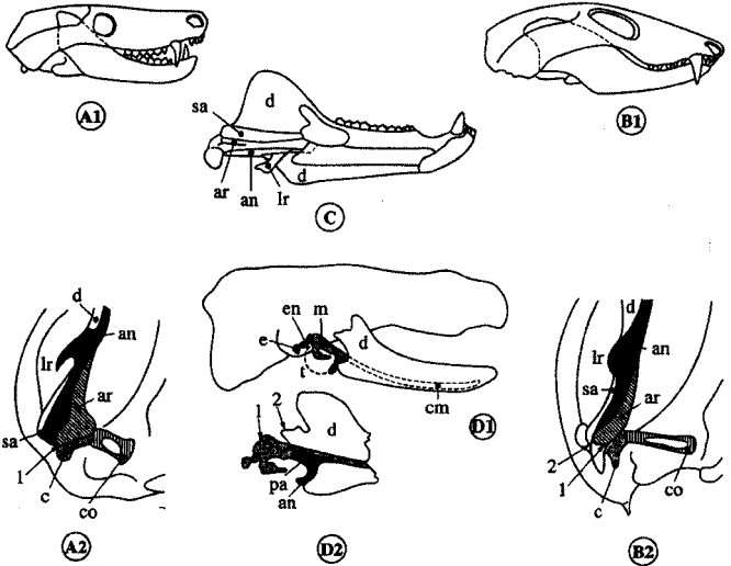
Şekil 49. A-B-C-Gelişmiş memeli sürüngelemlerin (Trias cynodontia'sı) kafatası yapısı. A1- Thrinaxodon ; ve A2-çene eklemelenmesi bölgesinde kafatasının iç görünümü. B1- Probainognathus ; ve B2-alt ve üst çene eklemelenmesini gösteren kafatasının iç görünümü, articularis ve kare arasında sürünge (1), yeni memeli (2), burada supra-angularis ve skuamosal arasında gerçekleşmiştir; diademodon 'un iç kısmından görülen çeneleri; lr, timpan halkası biçimi görünümünde angularisin parlak yüzü; keseli monodelphis 'in embriyo kafatası (3,5 mm.); D2-iç kısmından görülen çeneleri; cm, Meckel kıkırdağı; t, timpanın yeri; öteki kısaltmalar Şekil 47'deki gibi (A, B, Crompton'dan, C Watson'dan, D Maier'den alınmıştır; basitleştirilmiş biçimleriyle).
