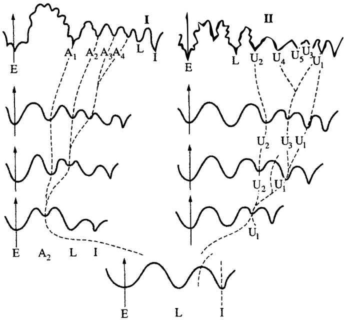
Şekil 38. Ammonitlerde bitişme çizgisinin gelişmesi. İlk başta sadece 3 protolob içeren [dış (E), yan (L) ve iç (I) (Alt Devoniyen'de anarcestidae)] bir desenden hareketle bitişme çizgisi ek loblarla yavaş yavaş karmaşıklaşmıştır. Bunlar dış ve yan loblar arasındaki çıkıntılar (I), ya da yan ve iç loblar arasındaki çıkıntıların (II) yarılmasıyla ortaya çıkarlar. Birinci süreç, ortaya çıkış sırasına göre doğuştan olmayan lobları verecektir (A1, A2, A3...). Esasen Paleozoik olan bu biçim goniatitina'nın belirgin özelliğidir. Kimi zaman, Üst Tebeşir döneminin seyrek rastlanan ammonitlerinde de görülür. İkinci süreç U göbek loblarını verir ve bunlar genel olarak kıvrımın bitişme çizgisinde bakışmı bir biçimde ortaya çıkarlar ve ortaya çıkış sıralarına göre numaralanmışlardır (U1, U2, U3). Paleozoikte çok ender görülen bu biçim sadece Permien'den sonraki dönemde yaygınlaşmıştır. Her iki olguda bitişme çizgisi daha sonra unsurlarının dekupajıyla karmaşıklaşabilir (değiştirilmiş biçimiyle Schindewolf'tan alınmıştır).
