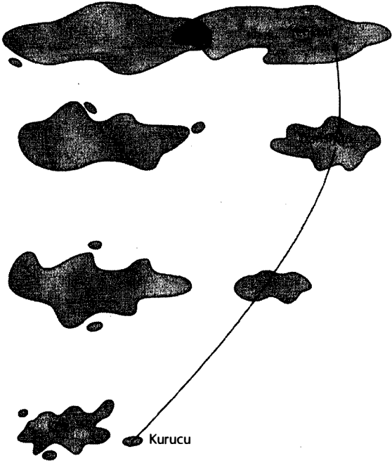
Şekil 23. Peripatrik türleşme modelinin ilke şeması: S-kök-topluluk; Kurucu, sonu ikincil olarak kökle ilişki kurabilen ama onunla meleleşemeyen yeni bir tür olan, gelişen bir genetiğin farklılaştığı yer (devrim).
