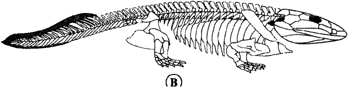
Şekil 29. A- Orta Devoniyen devri saçakyüzgeçlisi; B- Grönland'da Orta Devoniyen'de ilk kurbağagil ichthyostega . Solungaç kapağı öncesi ve solungaç kapağı (siyah), kuyruk yüzgeci, "balık"ta çok iyi gelişmiş yapılar kurbağagilde küçülmüş biçimde görülür (Jarvik'ten alınmıştır).
