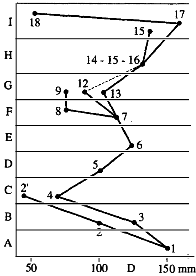
Şekil 1. Kosmoceras türü ammonitlerde olgun kabuğun boyunun değişmesi (Orta Jura Devri) [Tintant ve d.].
