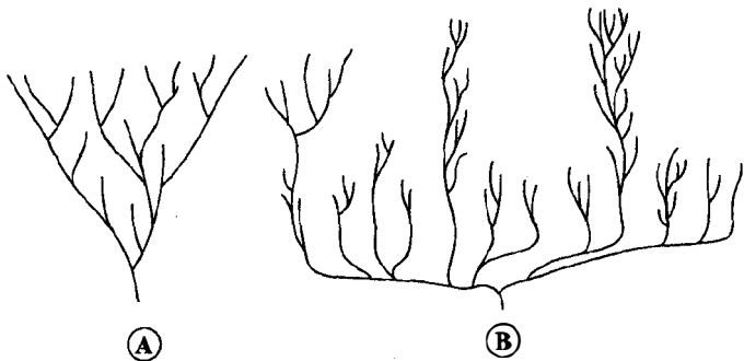
Şekil 34. İki evrim şeması: A- Klasik, artan çeşitlenme konisi görüntüsü; B- Biçimlerin ilk karmaşılaşması ve ardından çok az dal bırakan tahribat görüntüsü (Gould’dan alınmıştır).
