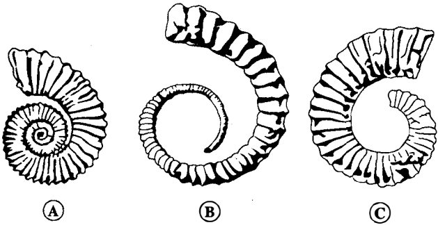
Şekil 39. Farklı ammonit gruplarında kavkının gelişmesinin ve görünümünün yinelenmeli dönüşümü: A- choristoceras (ceratitina, Üst Trias); spiroceras (ammonitina, Orta Jura Devri); crioceras (lyoceratina, Alt Tebeşir Devri) [Tintant'dan alınmıştır].
