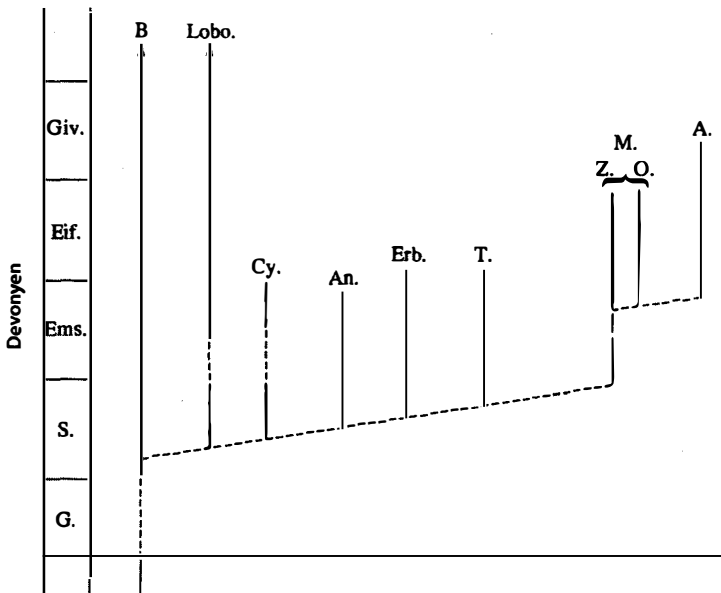
Şekil 36. Ammonitlerin kökeni. Aşağı Devonyen’de, dik kabuklu ve kavkılı ve karından sifonlu küçük orthoceras bactrites ’ten başlayarak önce eğimi gitgide artan kemerli bir dizi kabuklu biçim peşpeşe gelir ve sonunda sarmal kabuğa ulaşılır. Öte yandan bitişme çizgisi de bir dış lobun (R), daha sonra bir yan lobun (L) ve sonunda bir iç lobun (I) erken dönemde ortaya çıkışıyla karmaşıklaşır. Bu biçimlerin her biri, soyun daha sonraki evrelerinin ortaya çıkışından çok sonra uzun süre varolabilir. B- Bactrites ; Lobo- Lobobactrites ; Cy- Cyrtobactrites ; An- Anetoceras ; Erb- Erbenoceras ; T- Taicherteras ; M- Mimagoniantes ; A- Agoniantites (Wiedemann ve Erben den yararlanılarak düzenlenmiştir).
