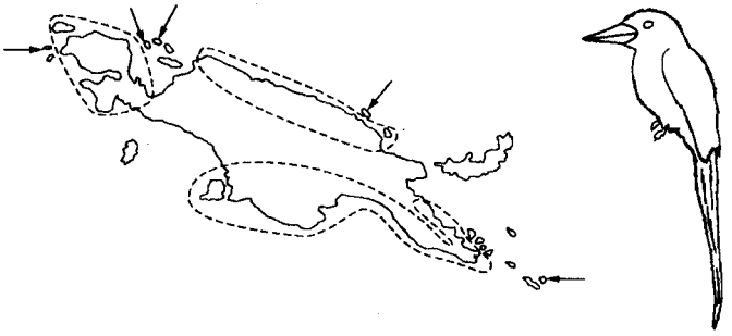
Şekil 22. Yeni Gine büyük adasında yalıçapkını tanyiptera galathea 'nın çok benzer (nokta nokta çizgiyle ayrılmış) üç biçimi vardır, buna karşılık komşu adalarda aynı türün farklı türler şeklinde tanımlanabilen oldukça farklı toplulukları (oklarla gösterilmiş) gelişmiştir (Mayr'den basitleştirilerek alınmıştır).
