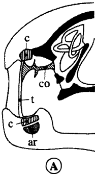
Şekil 48. Kulağın enine şematik kesitleri: A-Sürüngenin; B-Memelinin: ce, dış işitme borusu; co, Salyangoz; en, Örs kemiği; e, Üzengi; l, Sesleri alan salyangoz; m, Çekiç; t, Timpan; öteki kısaltmalar Şekil 47'deki gibi (basitleştirilmiş biçimiyle Goodrich'ten alınmıştır).
