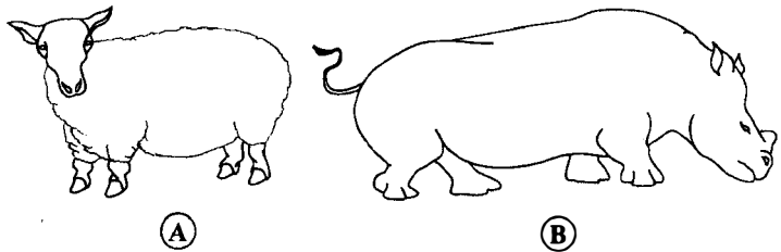
Şekil 27. A- Koyunun ancon (kısa bacaklı av köpeği) değişimi (Landauer'in bir fotoğrafından alınmıştır); B- Gergedan "kısa bacaklı av köpeği" Pliyosen'deki teleoceras (Ch. R. Knight'in bir tablosundan alınmıştır).
