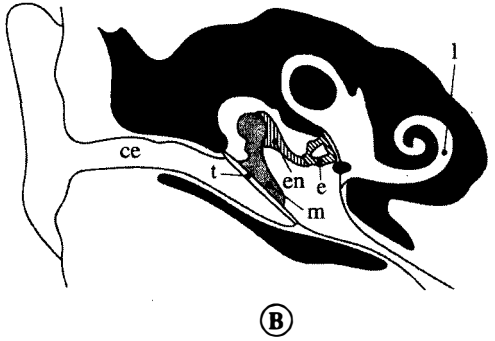
Şekil 48. Kulağın enine şematik kesitleri: A-Sürüngenin; B-Memelinin: ce, dış işitme borusu; co, Salyangoz; en, Örs kemiği; e, Üzengi; l, Sesleri alan salyangoz; m, Çekiç; t, Timpan; öteki kısaltmalar Şekil 47'deki gibi (basitleştirilmiş biçimiyle Goodrich'ten alınmıştır).
