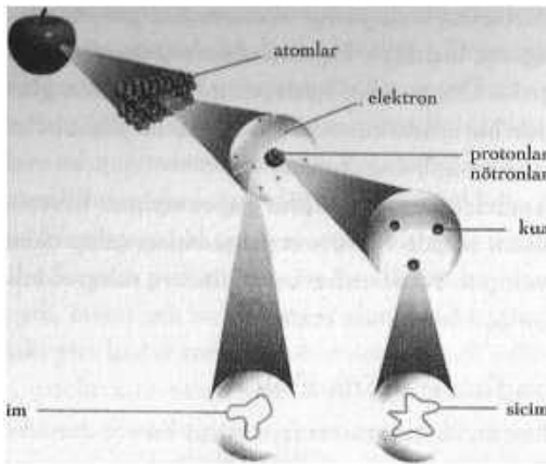
Şekil 1.1 Madde atomlardan oluşur, atomlar da kuarklar ve elektronlardan. Sicim kuramına göre, bütün bu parçacıklar aslında titreşen küçük sicim ilmekleridir.
