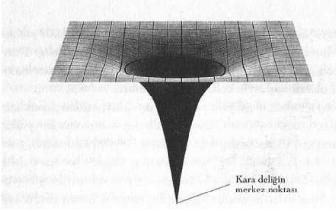
Şekil 3.7 Bir kara delik, etrafındaki uzay-zaman dokusunda o kadar ciddi bir yamulmaya sebep olur ki, "olay ufku" na -koyu renkli daireyle gösterilmiştir- giren hiçbir şey kara deliğin kütleçekiminden kaçamaz. Bir kara deliğin en derin noktasında tam olarak neler olduğunu hiç kimse bilmiyor.
