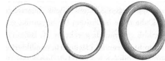
Şekil 12.8 Tip IIA sicim eşleşme sabiti artarken, sicimler tek boyutlu ilmeklerden genişleyip bir bisiklet tekerleğinin iç lastiğine benzer ikiboyutlu nesneler haline gelir.
