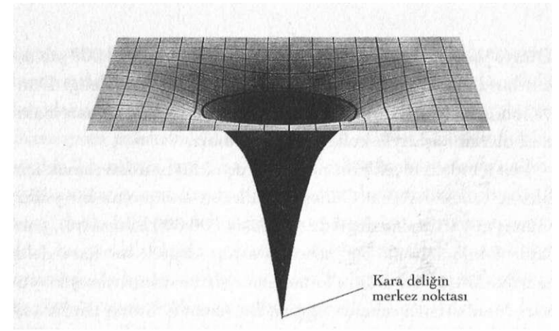
Şekil 3.7 Bir kara delik, etrafındaki uzay-zaman dokusunda o kadar ciddi bir yamulmaya sebep olur ki, "olay ufku"na -koyu renkli daireyle gösterilmiştir- giren hiçbir şey kara deliğin kütleçekiminden kaçamaz. Bir kara deliğin en derin noktasında tam olarak neler olduğunu hiç kimse bilmiyor.
