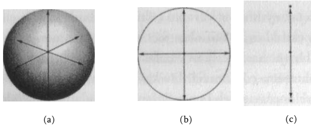
Şekil 13.2 Farklı boyutlardaki küreleri kolayca gözümüzde canlandırabiliriz; (a) iki, (b) tek ve (c) sıfır boyutlu küreler.
