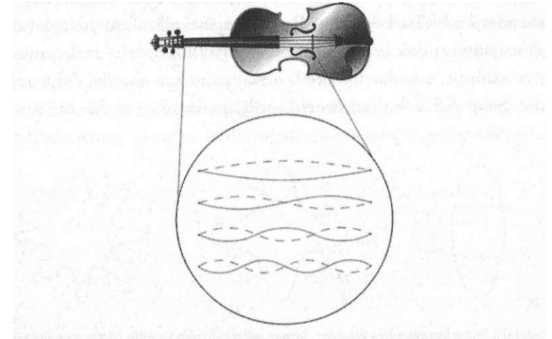
Şekil 6.1 Bir kemanın telleri, bütün tepe noktaları ve çukur noktaları keman telinin iki ucu arasına tam olarak oturan salınım örüntüleri sergileyerek titreşebilir.
