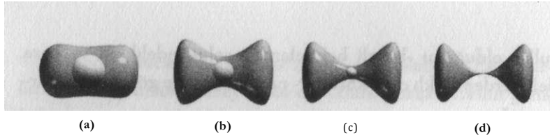
Şekil 11.3 Bir Calabi-Yau şeklinin içindeki küre bir noktaya kadar küçülür ve uzayın dokusunda bir sıkışmaya yaratır. Bunu ve sonraki şekilleri, Calabi-Yau şeklinin bir kısmını göstererek sadeleştirdik.
