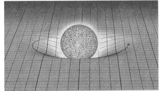
Şekil 3.5 Dünya Güneş'in çevresinde yörüngede kalır, çünkü yamulmuş uzay dokusundaki bir yol üzerinde ilerler. Daha açık bir ifadeyle, Güneş'in çevresindeki çarpılmış bölgede "en az direnç gösteren" yolu izler.
