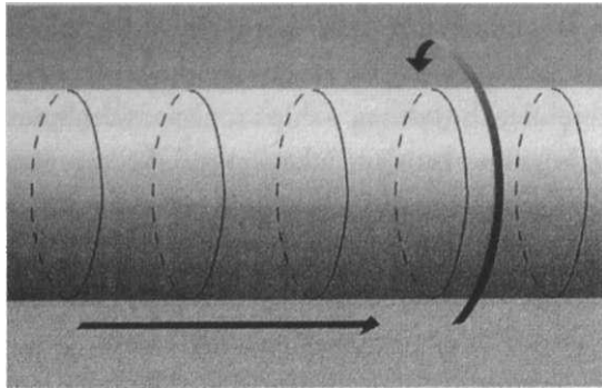
Şekil 8.2 Bahçe hortumunun yüzeyi ikiboyutludur. Boyutlardan düz okla gösterileni (yatay yay ılımı) uzun ve uzamıştır; dairesel okla gösterilen diğ er boyut ise (daire sel çevresi) kısa ve kıvrılmıştır.
