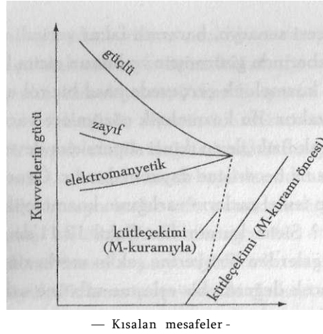
Şekil 14.2 M-kuramı çerçevesinde, dört kuvvetin güçleri doğal olarak birleşebilir.
