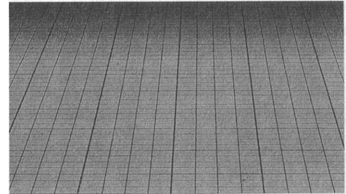
Şekil 3.3 Düz uzayın şematik bir temsili
