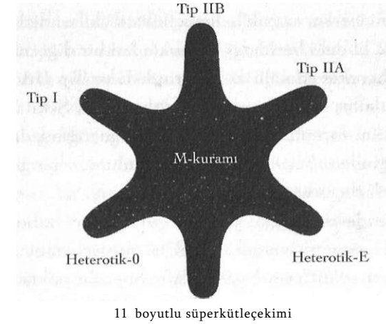
Şekil 12.1 1 İkiliklerin dahil edilmesiyle birlikte, beş sicim kuramı, 11 boyutlu süperkütçekimi ve M-kuramı birleşik bir çerçevede bir araya getirildi.
