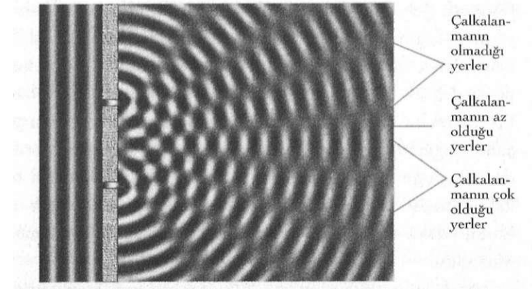
Şekil 4.7 Deliklerin her birinden çıkan dairesel su dalgaları üst üste biner, bu da toplam dalganın bazı yerlerde büyümesine bazı yerlerde küçülmesine yol açar.
