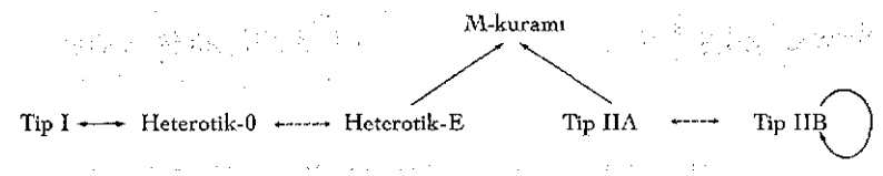
Şekil 12.10 Beş sicim kuramı ve M-kuramı uzay-zamanın geometrik biçimini (X. Bölüm'de olduğu gibi) gerektiren ikilikleri içererek, bir ikilikler ağıyla birleşir.
