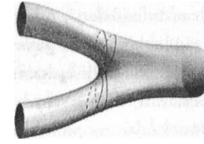
Şekil 6.10 George ile Gracie, iki sicim arasındaki etkileşimin yeri konusunda anlaşamaz.
