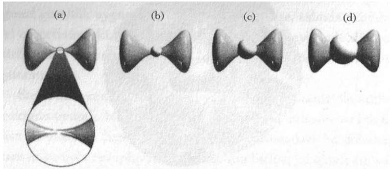
Şekil 11.4 Sıkışmış bir Calabi-Yau şekli yırtılır ve bu noktada yüzeyi düzelten bir küre gelişir. Şekil 11.3'teki ilk küre "sönmiştir".
