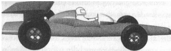
Şekil 2.4 Hareket eden bir nesne hareket doğrultusunda kısalır.
