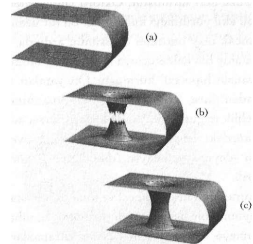
Şekil 11.1 (a) "U şeklindeki" bir evrende, bir uçtan diğer uca gitmenin tek yolu evrenin tamamını kat etmektir, (b) Uzayın dokusu yırtılır ve bir solucandeliğinin iki ucu belir-meye başlar, (c) İki uç birleşir ve evrenin bir ucundan diğerine uzanan yeni bir köprü -bir kestirme yol- oluşur.
