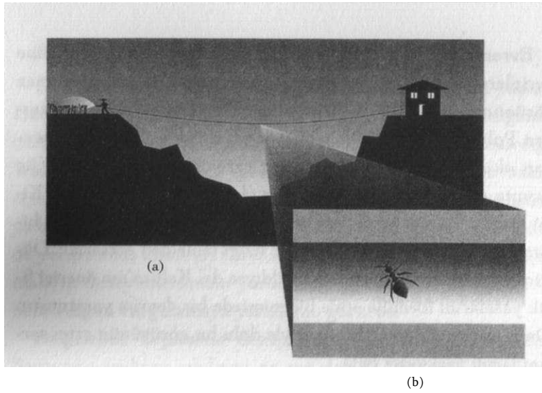
Şekil 8.1 (a) Epey uzak bir mesafeden görülen bir bahçe hortumu, tek boyutlu bir nesne gibi görünür, (b) Bu görünüm büyütüldüğünde, bir daire şeklinde hortumun çevresini saran ikinci bir boyut görünür hale gelir.
