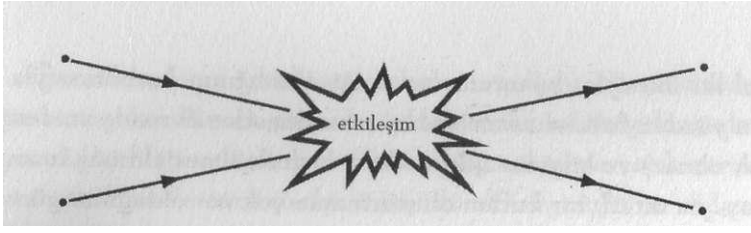
Şekil 6.5 İki parçacık etkileşime girer -birbirleriyle "çarpışır"- ve bunun sonucunda ikisinin de izlediği yol değişir.
