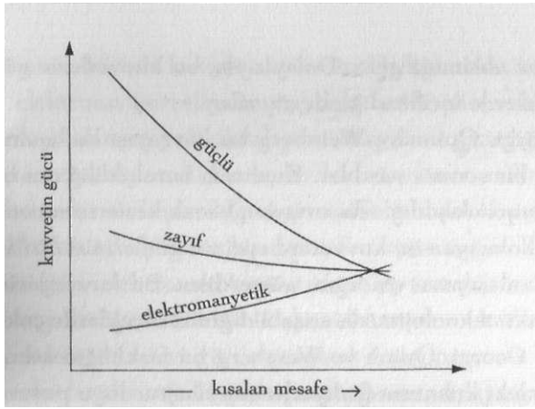
Şekil 7.1 Kütleçekimsel olmayan üç kuvvetin, giderek kısalan mesafe ölçeklerinde (buna eşdeğer olarak giderek yükselen enerji süreçlerinde) hareket ederkenki güçleri
