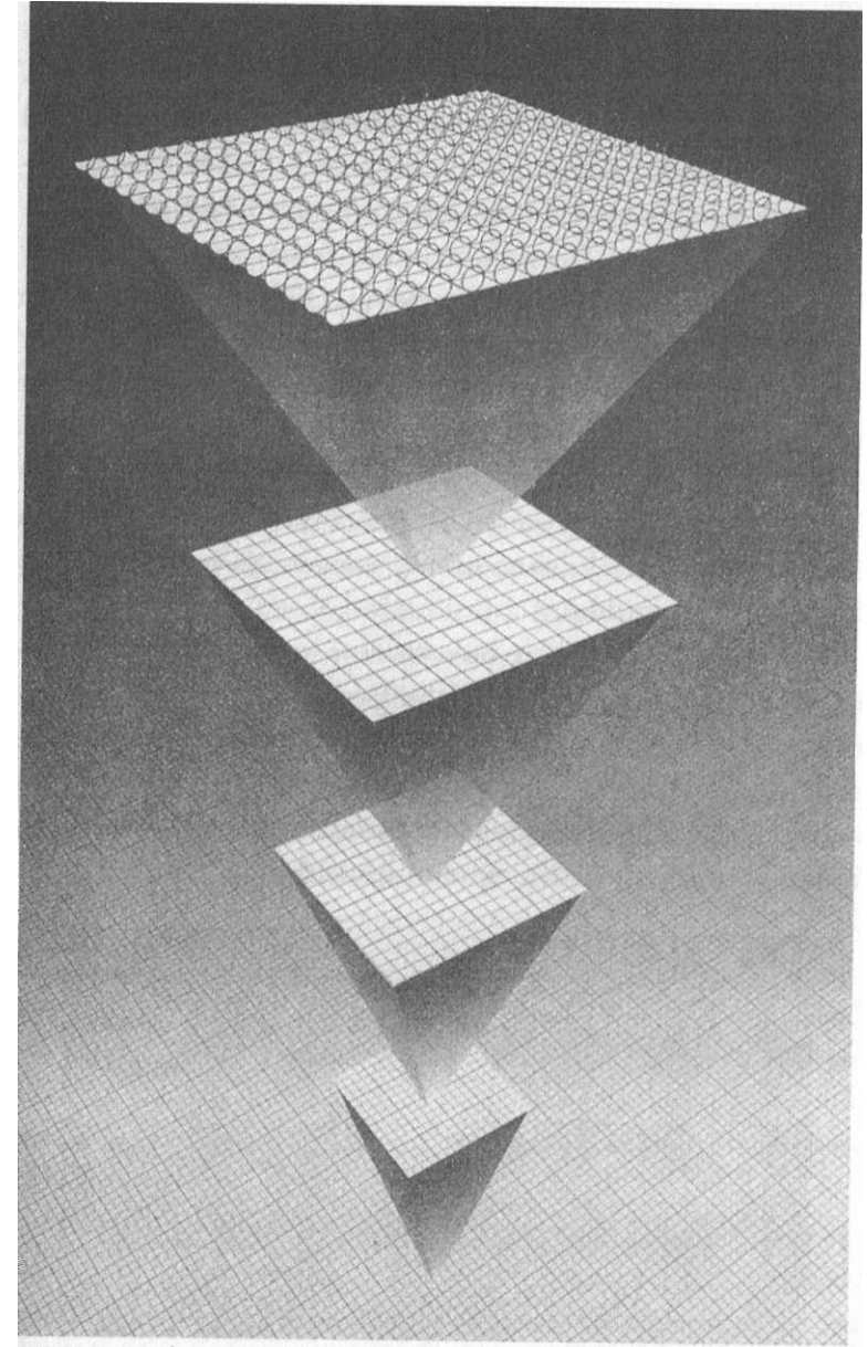
Şekil 8.3 Şekil 5.1'de olduğu gibi, birbirini izleyen her kademe, bir önceki kademe de gösterilen uzamsal dokunun devasa boyutlarda büyültülmüş halini temsil etmektedir. Büyültmenin dördüncü aşamasında gördüğümüz gibi, bugüne kadar doğrudan gözlenememiş olmaları sonucunu doğuracak kadar küçük bir uzayda kıvrılmış olmaları koşu- luyla, evrenimizde başka boyutlar da olabilir.
