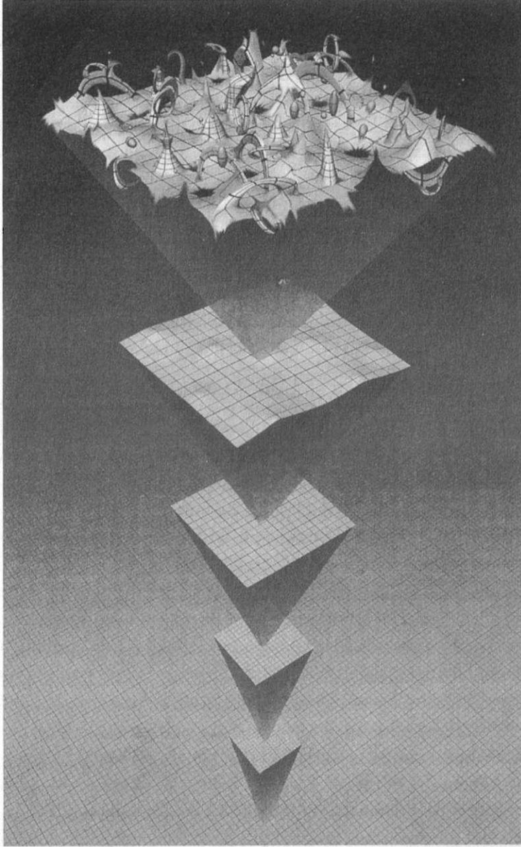
Şekil 5.1 Uzayın bir bölgesini aşama aşama büyütürük, ultramikroskobik özelliklerini inceleyebiliriz. Genel görelilik ile kuantum mekaniğini birleştirme girişimleri, büyütmenin en son aşamasında ortaya çıkan şiddetli kuantum dalgalanmalarına ters düşmektedir.
