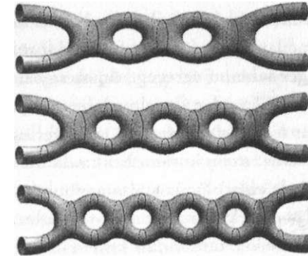
Şekil 12.5 Kuantum çığnlığı, çok sayıda sicim/antisicim çifti dizisinin ortaya çıkması ve ortadan kalkmasına neden olabilir.
