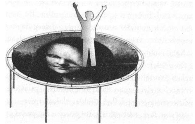
Şekil 10.1 Mona Lisa trampolini üzerinde dururken, görüntü en çok vücudunuzun ağırlığı altındaki kısımda çarpılır.
