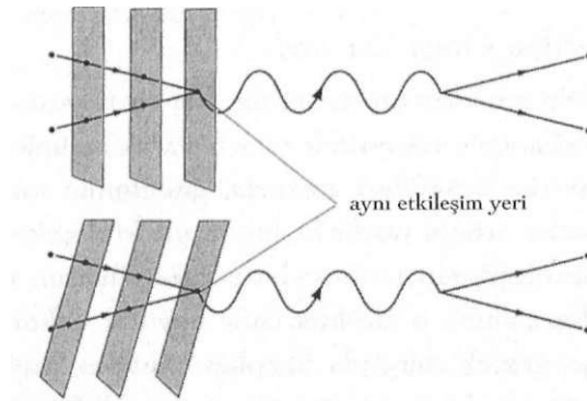
Şekil 6.11 Göreli hareket halindeki gözlemciler, iki nokta parçacığın birbirleriyle ne zaman ve nerede etkileştiği konusunda anlaşmaz.
