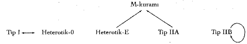
Şekil 12.9 Oklar, hangi kuramların birbiriyle ikilik oluşturduğunu göstermektedir.
