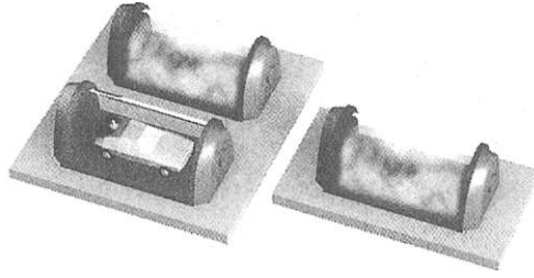
Şekil 15.1 Tele-taşımaya hayalci bir yaklaşım, birbirlerinden uzakta olan ve kuantum dolanık parçacıklarla dolu iki odayı ve tele-taşınacak cismi oluşturan parçacıklarla birlikte odalardan birindeki parçacıkları aynı anda ölçebilecek bir aracı göz önüne alır. Bu ölçümlerin sonucu, daha sonra ikinci odadaki parçacıkları cismi kopyalayacak şekilde değiştirmek ve tele-taşımayı sonuçlandırmak için gerekli olan bilgileri sağlar.
