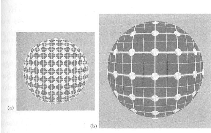
Şekil 8.2 (a) Eger bir kürenin yüzeyine eşit aralıklarla bozuk paralar yapıştırılırsa, herhangi bir paradan görülen manzara diğeriyle aynıdır. Bu da herhangi bir galaksiden bakıldığında görülenlerin, bir başka galaksiden bakıldığında görüleceklerle aynı olduğu yolundaki inancımızla örtüşür. (b) Eger küre genişlerse, paralar arasındaki uzaklık artar. Üstelik, 8.2a'daki iki para birbirinden ne kadar uzaksa, 8.2b'deki genişleme sırasında da aralarındaki uzaklık o kadar çok artar. Bu da bir galaksiye bakılan nokta ne kadar uzak olursa, galaksinin o noktadan o kadar hızlı uzaklaştığı yolundaki ölçümlerimizle paralellik gösterir. Dikkat ederseniz, burada hiçbir para, özel olarak diğerlerinden ayrılmaz ki bu da evrendeki hiçbir galaksinin uzayın genişlemesinin merkezi veya özel bir noktası olmadığı inancımızı destekler.
