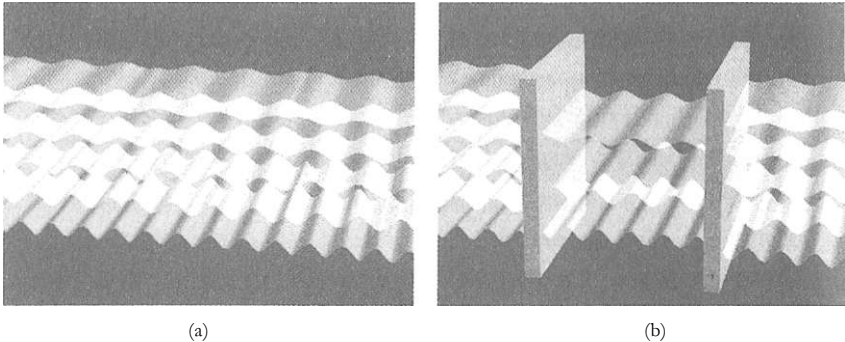
Şekil 12.1 (a) Elektromanyetik alanın boşluk titrenimleri (b) İki plakanın arasındaki boşluk titrenimleri
