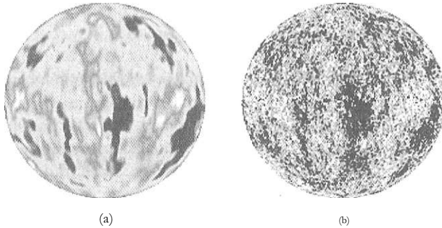
Şekil 14.4 (a) COBE uydusu tarafından toplanan kozmik mikrodalga fon ışıyım verileri. Bu ışıyım, Büyük Patlama'nın yaklaşık 300.000 yıl sonrasında beri Hiçbir engelle karşılaşmadan yayılıyor, o yüzden bu şekil, evrende hemen hemen 14 milyar yıl önce var olan sıcaklık farklılıklarını gösteriyor, (b) WMAP uydusu tarafından toplanan geliştirilmiş veriler
