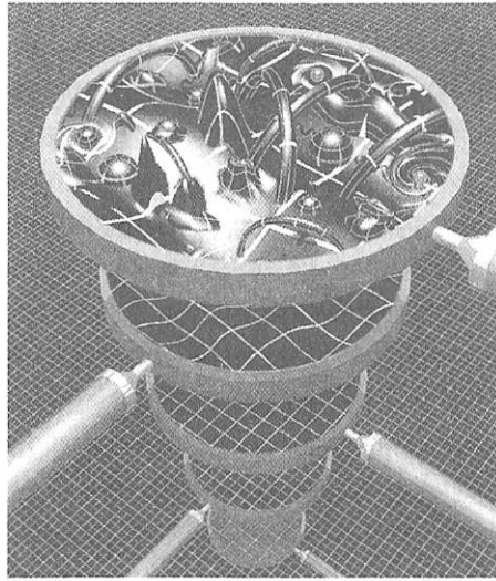
Şekil 12.2 Uzayın ardışık büyötmeleri, Planck uzunluğunun altında uzayın kuantum titrenimleri nedeniyle tanınamayacak kadar karmaşık olduğunu ortaya koyar. (Bunlar, her biri 10 milyon ile 100 milyon kez arasında büyötmeye sağılayan hayali büyöteçlerdir.)
