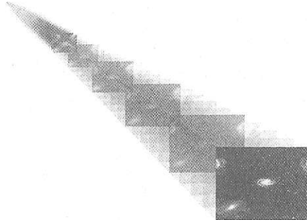
Şekil 8.10 Düz ve sonlu boyutlu olan bir evrenin kozmik geçmişi; uzay-zaman "somunu". Tepedeki bulanıklık, evrenin başlangıç dönemindeki kavrayışımızın eksikliğini simgeliyor.
