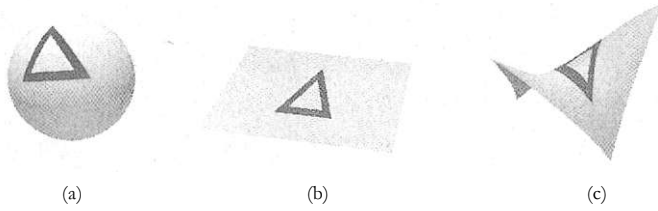
Şekil 8.6 Uzunluk için iki boyutlu benzetmeler kullanırsak, tam anlamıyla simetrik olan -yani biryerden görülen manzaranın diğer yerlerde görülenlerle aynı olduğu- üç tür eğrilik vardır. Bunlar (a) kürede olduğu gibi, dışarı doğru bir örnek şişen pozitif eğrilik; (b) sonsuz bir düzlem veya sonlu video oyunu ekranındaki gibi, hiç şişmeyen sıfır eğrilik; (c) eyer şeklinde olduğu gibi, içeri doğru bir örnek büzülen negatif eğrilik.
