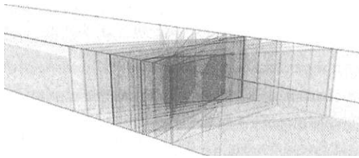
Şekil 5.5 Dünya dan değişik uzaklıklarda bulunan ve değişik hızlarla hareket eden çeşitli gözlemciler için (gerçek ya da hayali) zaman dilimleri örneği
