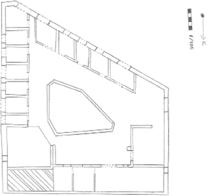
Işık Hamamı Üst Kat Planı (Eskişehir Vakıflar Şube Müdürlüğü)
