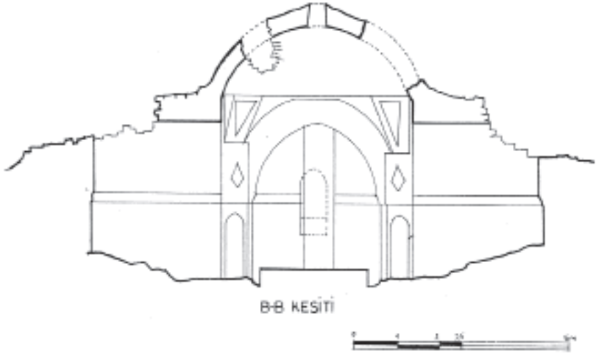
Seyidiler Hamamı B-B Kesiti(Erol Altınsapan, Sivrihisar'da Türk Mimarisi, Selçuk Üniversitesi Sosyal Bilimler Enstitüsü Yayınlanmamış Yüksek Lisans Tezi, Konya, 1988)
