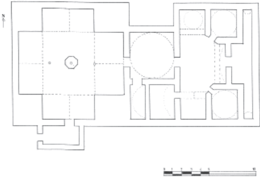
Kumacık Hamamı Rölöve Planı (Erol Altunsapan, Sivrihisar'da Türk Mimarisi, Selçuk Üniversitesi Sosyal Bilimler Enstitüsü Yayınlanmamış Yüksek Lisans Tezi, Konya, 1988)
