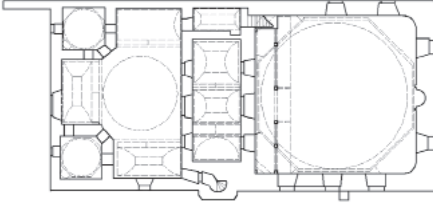
Ak Camii Rölöve Planı ( Soner Uğurlu 2007'den ilavelerle)
