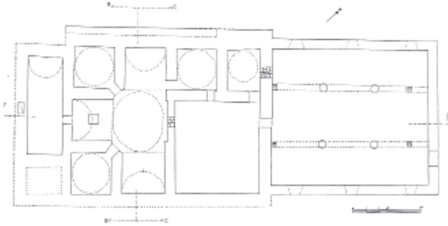
Seyidiler Hamamı Rölöve Planı(Erol Altınsapan, Sivrihisar'da Türk Mimarisi, Selçuk Üniversitesi Sosyal Bilimler Enstitüsü Yayınlanmamış Yüksek Lisans Tezi, Konya, 1988)
