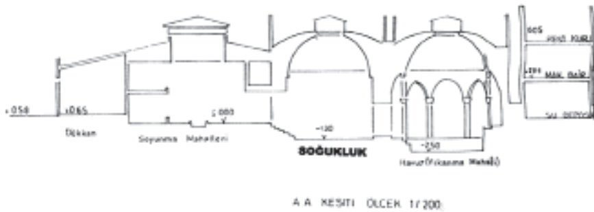
Erler Hamamı A-A Kesiti(Eskişehir Vakıflar Şube Müdürlüğü)
