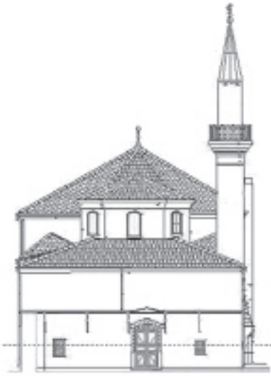
Kuzey Cephe Rölövesi ( Baha Yiğit, 2007)
