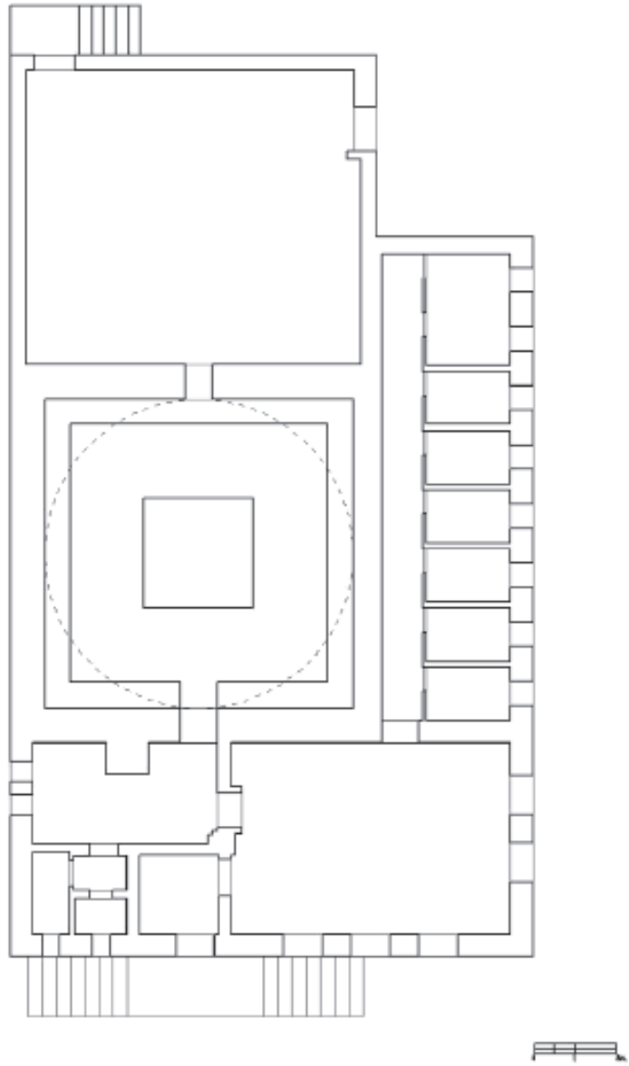
Mihalıççık Belediye Hamamı Rölöve Planı (Rölöve: Ali Gerengi, Bülent Okta, H. Berkant Özdemir Çizim: Ali Gerengi)
