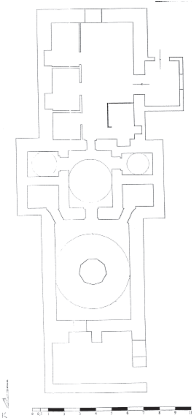
Mahmudiye Hara Hamamı Rölöve Planı
