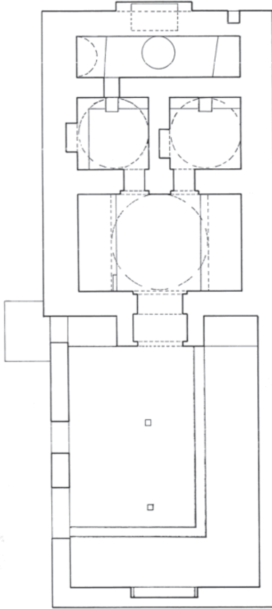
Han Hamamı (Hüsrev Paşa Hamamı) Rölöve Planı (Tuncay Arslantekin, Mevlüt Erbaş, Ahmet Ofu, Feyza Oğultekin, Gülgün Örsel, Betül Pekmez, “Han Bölgesi, Türk Dönemi Yapıları”, Anadolu Üniversitesi Edebiyat Fakültesi Sanat Tarihi Bölümü, 1999 yılında Öğr. Gör. Abdullah DEVECİ danışmanlığında bitirme ödevi olarak hazırlanan çalışmadan alınmıştır.)
