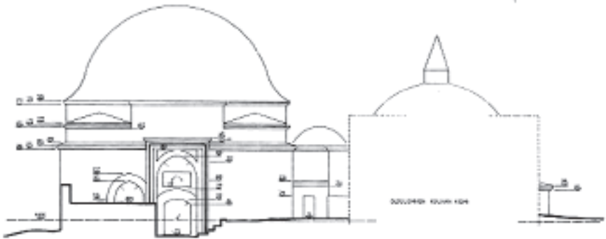
Seyitgazi Selçuk Hamamı Doğu Cephe(Eskişehir Vakıflar Şube Müdürlüğü)
