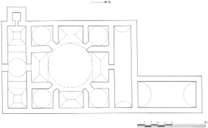
Gavur Hamamı Rölöve Planı (Erol Altınsapan, Sivrihisar’da Türk Mimarisi, Selçuk Üniversitesi Sosyal Bilimler Enstitüsü Yayınlanmamış Yüksek Lisans Tezi, Konya 1988)
