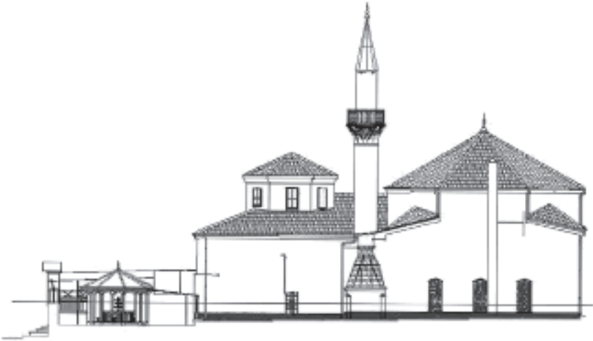
Batı Cephe Rölövesi ( Baha Yiğit, 2007)
