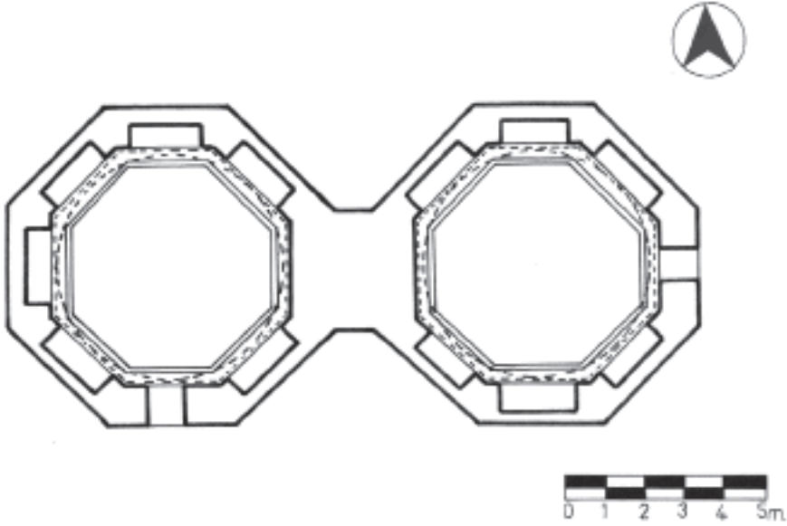
Hamam Karahisar köyü Çardak Hamamı Rölöve Planı (E.Altınsapan-C. Parla, Eskişehir Selçuklu ve Osmanlı Yapıları I, Anadolu Üniversitesi Yayınları Eskişehir 2004)
