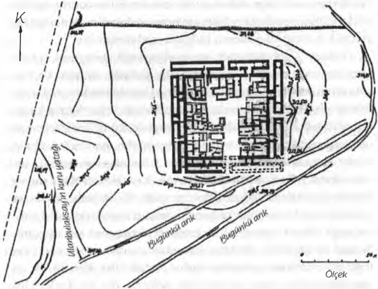
Şekil 6.26. Sapalı Tepe (Sarianidi).
