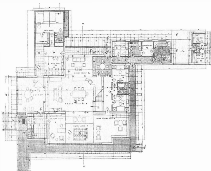
Resim 1: Çankaya'da Bir Villa, Seyfi Arkan. ( Arkitekt 1936, n. 7, ss. 179-186)
