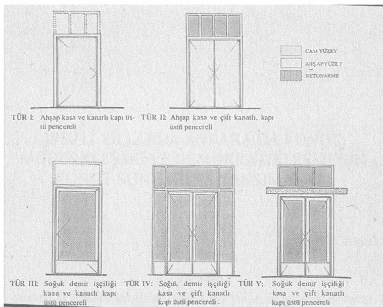
Resim 5: Kapı üstü pencerelerinin kapı üzerinde yerleşimleri. (Kaprol 2000: 197)
