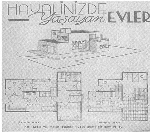
Resim 2: Dönemin popüler yayını Yedigün 'de yeni yaşam biçimini öneren konutlar ve yerleşim planlarına sık sık yer verilmekteydi. (Anon. 1934)
