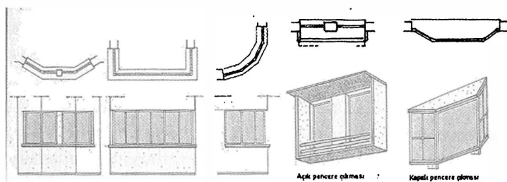
Resim 6: Yatay nispetli pencere, köşe penceresi, açık ve kapalı pencere çıkması. (Kaprol 2000: 204)
