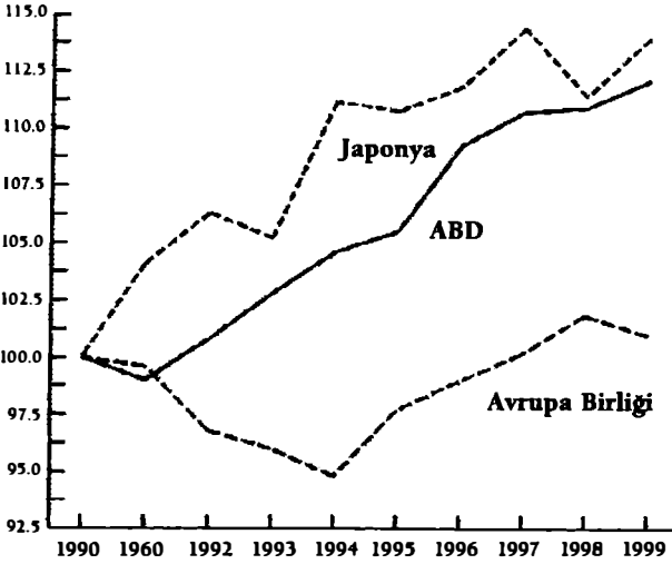
Şekil 1: 1990'larda Karbon Dioksit Emisyonlarındaki Değişiklikler (1990 = 100)
