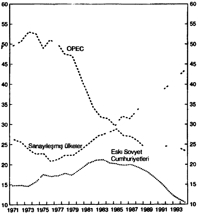
Şekil 2. Ülke Gruplarına Göre Petrol Arzı (yüzde olarak)
