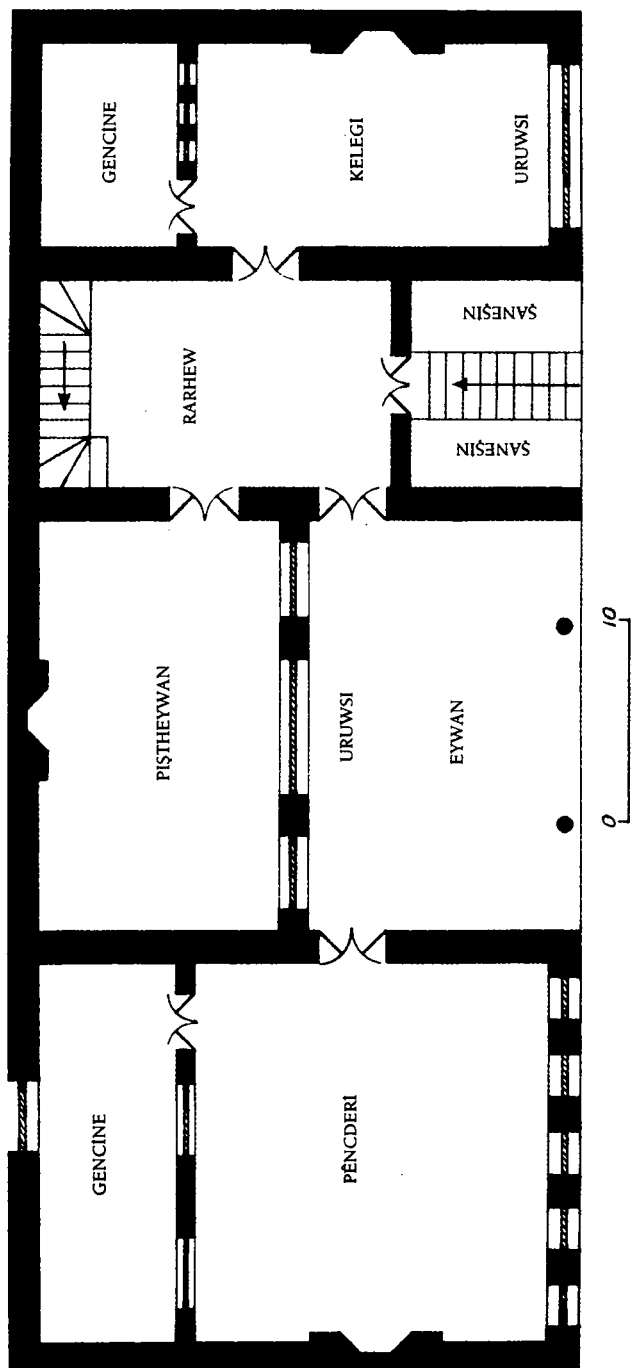
Figür 1. Bir Kürt kent evinin planı. Birinci kat. Ölçek yaklaşık 1: 100
