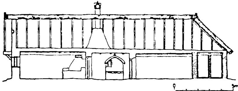
Yukarıdaki evin yan kesiti
