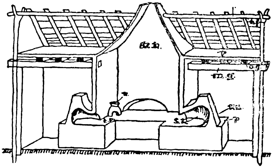
Şekil 1. Ortasında mutfak ve her iki yanında ısıtılmış odalar bulunan üç bölümlü Macar evi
