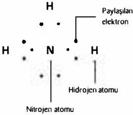
Kovalent bağlar
