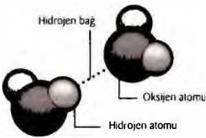
Hidrojen bağlar
