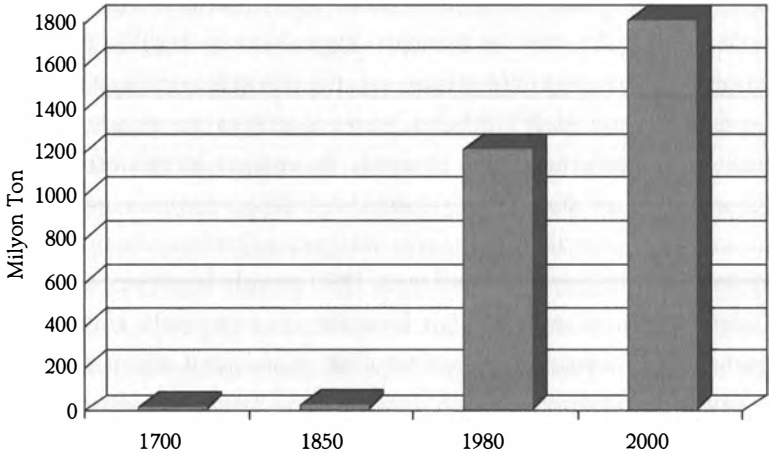
Dünya genelinde demir-çelik üretimi, 1700-2000
