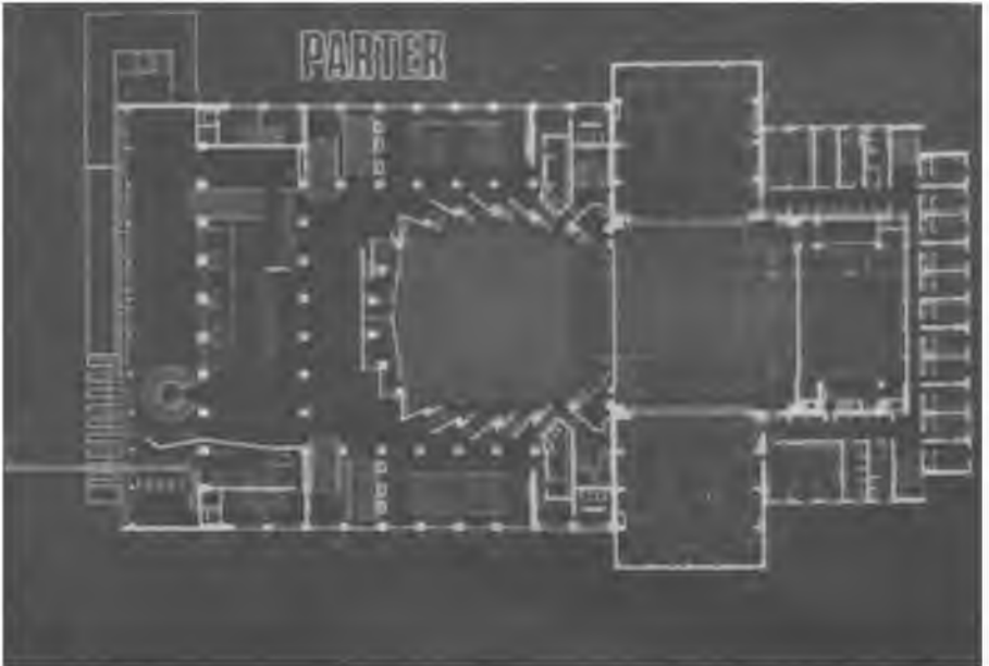
Resim 91: Temeli 1947'de atılan, 1969'da tamamlanan, 1970 yılının sonunda yanan ve sonra tekrar yapılarak 1973'de halka açılan İstanbul Atatürk Kültür Merkezi'ndeki büyük tiyatronun planı.
