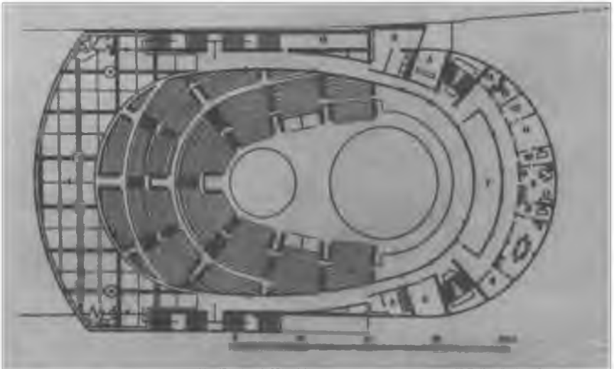
Resim 28: Meyerhold'un yaptırdığı tiyatronun 1932'deki planı. Mimarları Mikhail Barkhin ve Sergei Vakhtangov'tur. (E. Braun)
