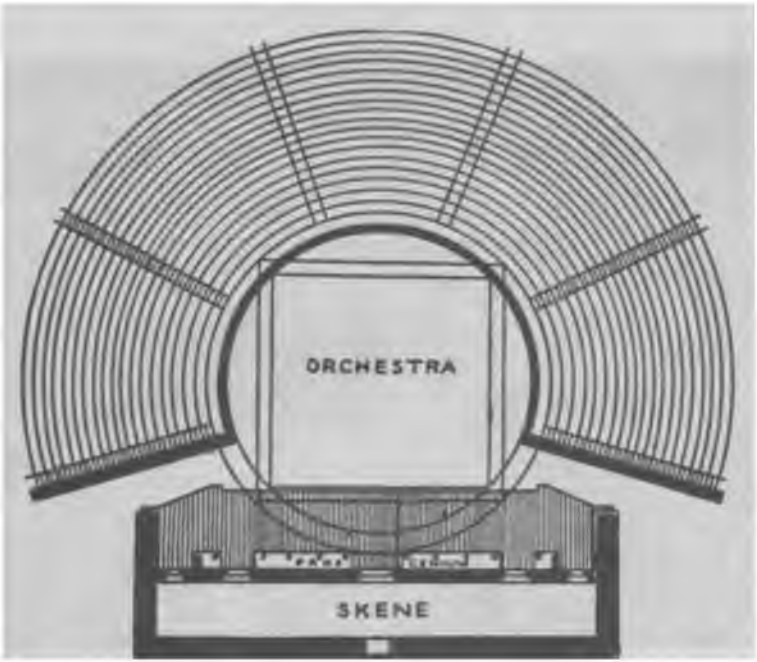
Resim 10: Roma Dönemi Tiyatro plânı: Termessos - Burdur. (Flickinger)
