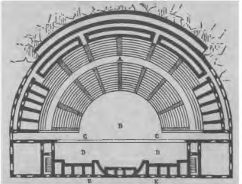
Resim 13: Roma Tiyatrosu Plânı. (Margarete Bieber)
