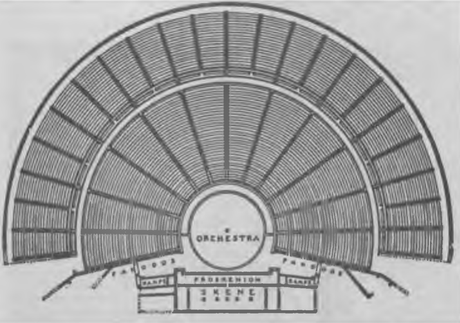
Resim 7: Hellenistik Dönem Yunan Tiyatrosu (Dörpfeld-Reisch'tan)
