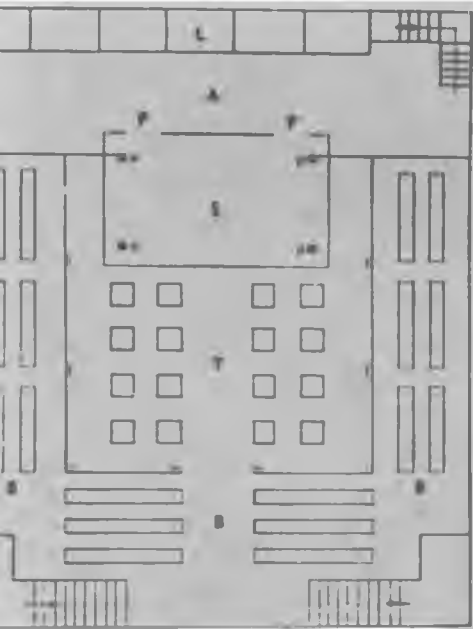
Resim 49: Klâsik Çin Tiyatrosu oyun yeri: L — oyuncuların giyinme odaları, A — Oyuncuların dinlenme salonu, P — Giriş (soldaki) ve çıkış (sağdaki) S — Sahne, T — İmtiyazlı kişilere ayrılan yerler, B — Yandaki ve gerideki sıralar.
