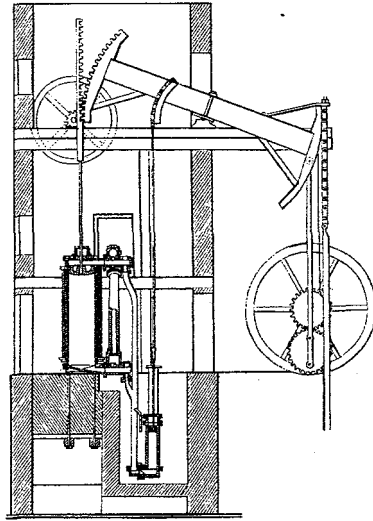
Watt'ın çift etkili buhar makinesi, 1769.
