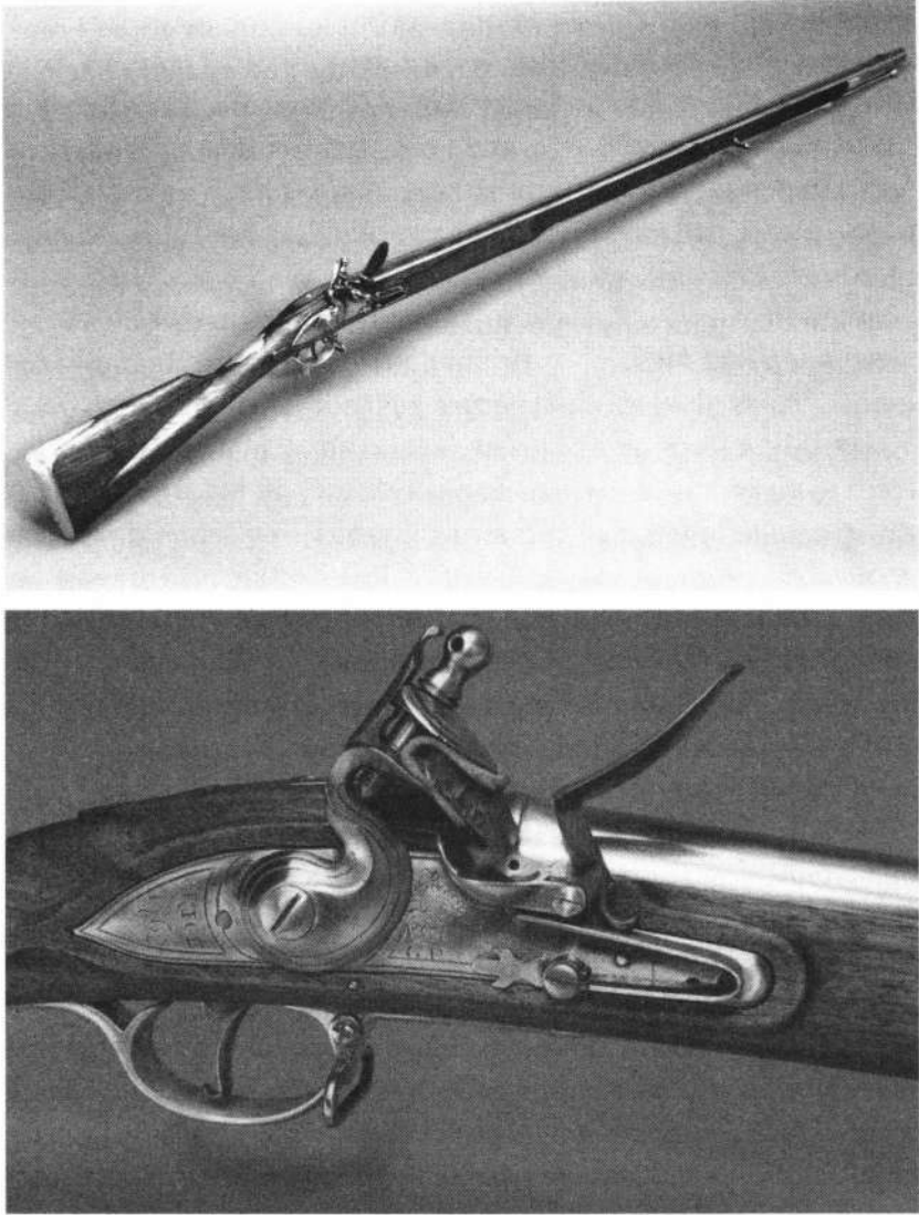
Resim 8.1 Fransız filintasının iki açıdan görünümü (Kraliyet Topçu Bölüğü, Quebec).
