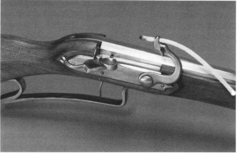
Resim 6.3 Fitilli tüfek mekanizmasına yakından bakış (Kraliyet Topçu Bölüğü, Quebec).
