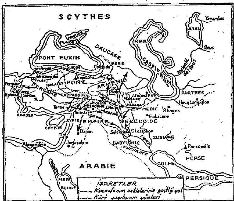
HARİTA I. - İlkçağda Kürtler
