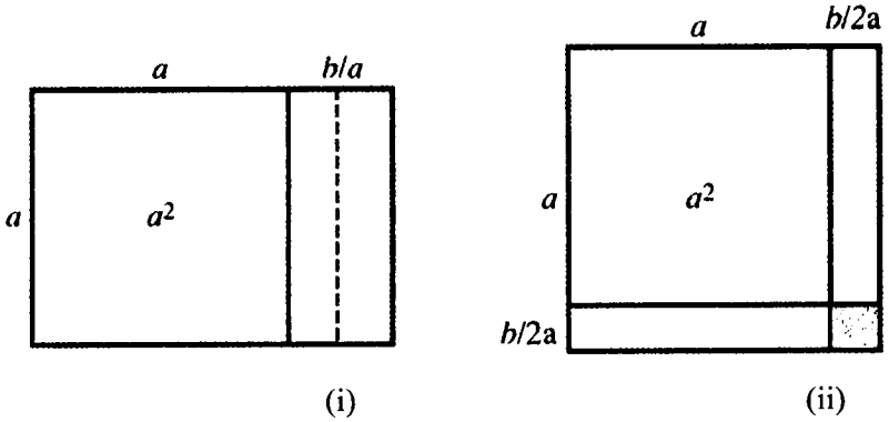
Şekil 11: (i) a alanı ile b alanının gösterimi (ii) ikiye bölünen b alanın yeni konumu.
