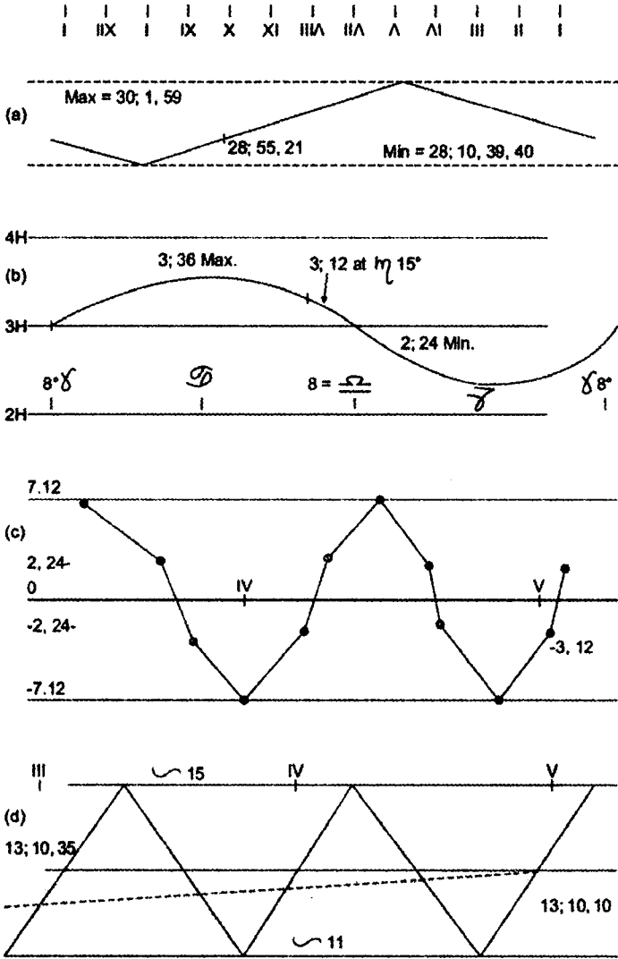
Şekil 13: (a) Her ay için Güneş hızının hesaplanan yaklaşık değeri (b) Kavuşum konumunda gün uzunluğu (c) Ay'ın Güneş yörüngesinin altında ve üstündeki enlem değeri (d) Kavuşum konumunda Güneşin hızı
