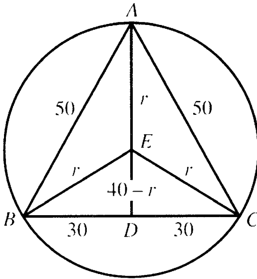
Şekil 9: Pisagor bağıntısı kullanılarak çember içine çizilmiş üçgenin kenar uzunluklarına bağlı yarıçapı bulma problemi.
