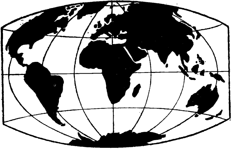
Yerküresinin Karaparçalarının Bugünkü Durumları
