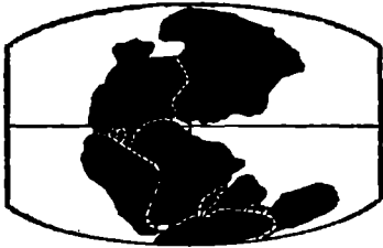
Yerküresinin Karaparçalarının 200 Mil. Yıl Önceki Durumları.
