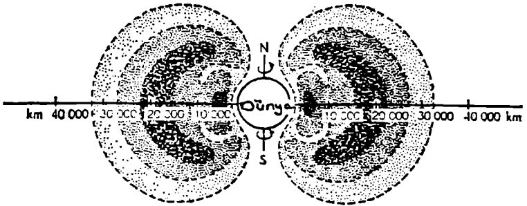
Yerküresinin manyetik alanı ve uzaydaki dağılımı. (Malachow'dan s. 105)
