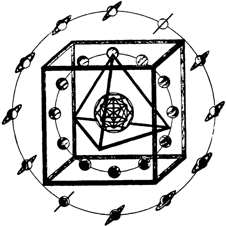
Resim 35. — Satürn, Jüpiter ve Mars'ın yörüngeleri.
