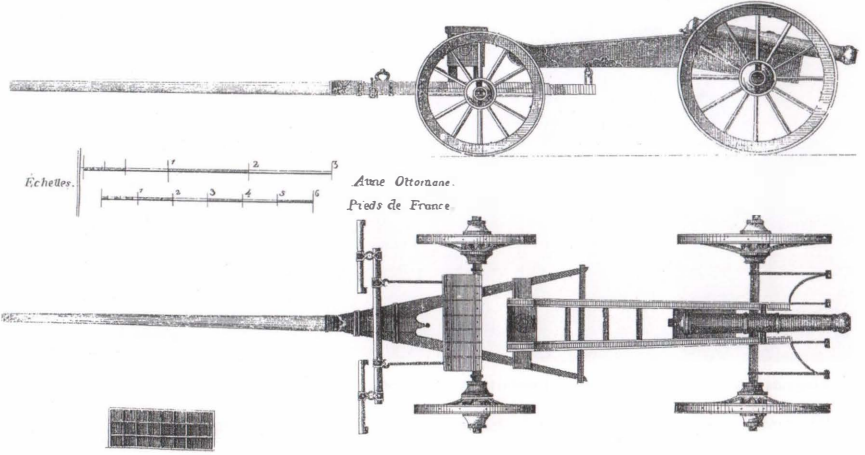
Fransız maceracı Baron de Tott'un danışmanlığında 1774'te kurulan Sûret Topçuları Ocağı, bu güzel plan gravüründe tasvir edilen tarz çabuk doldurulup ateşlenen ve muharebede sürekli yer değiştiren seyyar toplar kullanmak üzere talim görüyordu (Mahmud Râif Efendi).
