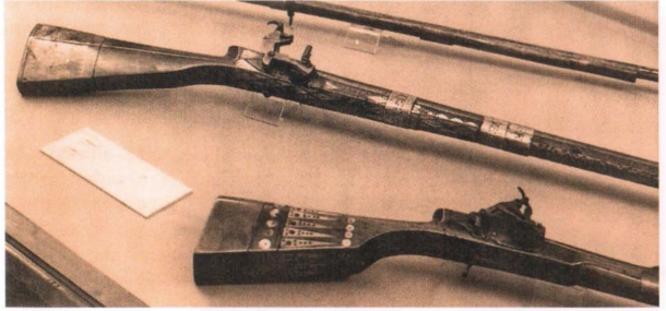
18. yüzyıl sonlarından kalma çakmaklı Türk tüfekleri. Mekanizma basit ve alabildiğine dayanıklıdır; daha önceki fitilli tüfeklerde olduğu gibi, tetiğe kazara basılmasını engelleyen muhafazalar yoktur (Yazarın fotoğrafı, Harbiye Askeri Müzesi, İstanbul).
