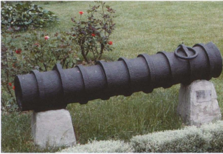
Bu Memlük yahut Osmanlı topu, 15. yüzyıl sonlarına tarihlendirilir. Dövme demir kasnakların yine dövme demirden çemberlerle tutturulmasıyla yapılmıştır (Askeri Müze, İstanbul; yazarın fotoğrafı).
