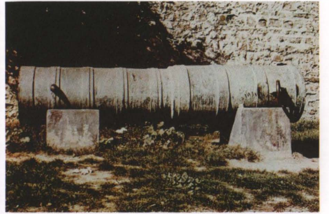
Bu Osmanlı topu, 15. yüzyıla ait pek çok resimde görülen türdendir. Dar barut haznelidir ve tunçtan mamuldür (Askeri Müze, İstanbul).
