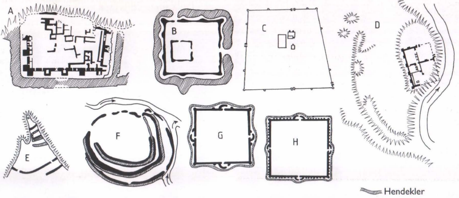
Tahkimatlar: A- İgduy Kale, Harezm, 4-5. yüzyıl (Tolstov'dan) B- Uygur hisarı, Tuva bölgesi, 8-9. yüzyıl (Pletnyeva'dan) C- Pliska iç-kalesi, Bulgaristan, 8-9. yüzyıl (Rashev'den); D- Alan-Hazar dönemi hisarı, Dağıstan, 8-10. yüzyıl (Pletnyeva'dan); E- Bir tepenin ucu-na kurulu hisar, Kuzey Kafkaslar, 9-13. yüzyıl (Pletnyeva'dan); F- İdil Bulgarlarına ait bir hisar, 10-12. yüzyıl (Pletnyeva'dan); G-H- Amur Nehri bölgesindeki küçük ve büyük kaleler, 10-13. yüzyıl (Derevyanko'dan).
