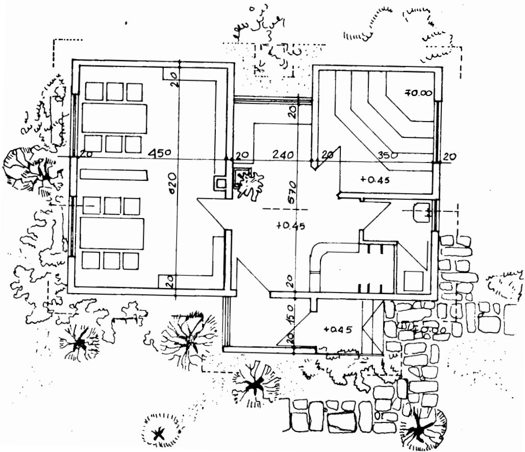
Köy kitaplığı için plan : İnşaat mühendisi mimar Orhan Özbay
