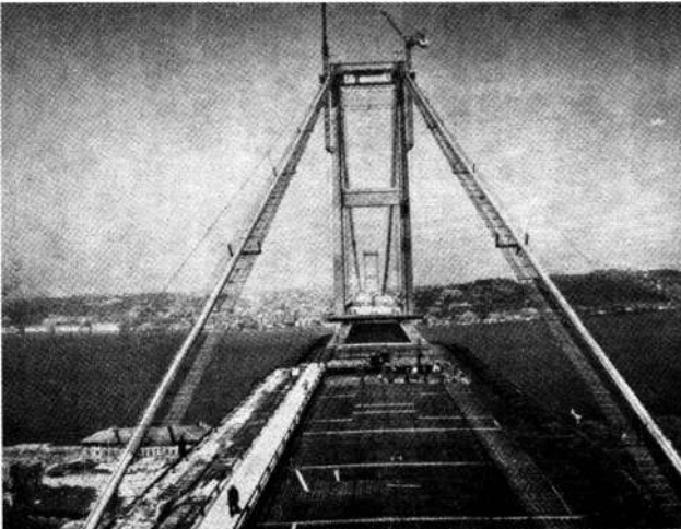
Üçüncü Haliç Köprüsü İnşaatı
