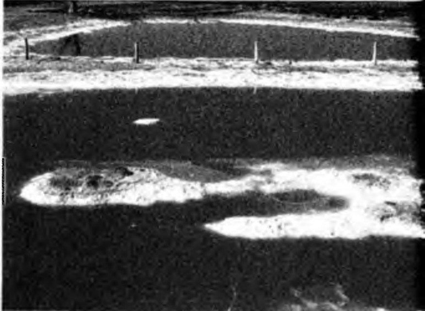
Resim 28. Avusturalya'nın en büyük nehri olan Murray Nehri boyunca gözlemlenen bir tür tuzlulaşma şekli olan yüzeydeki tuz birikintileri.
