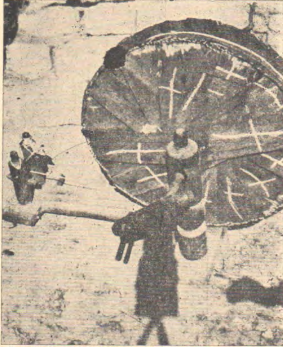
Resim 2: ÇIKRIK. Eğrilmiş olan yun ipini daha ziyade bükmek veyahut iki ipi bir araya getirip kalın ip yapmak için kullanılan bir alettir.
