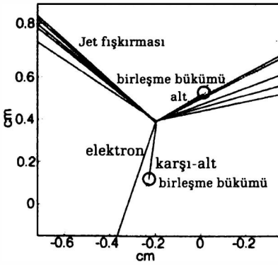
ŞEKİL 43 Alt kuarklardan oluşan hadronlar diğer yüklü parçacıklara bozunmadan önce dedektörde görülebilir bir iz bırakacak kadar uzun yaşarlar. Bu, silisyum tepe dedektörlerinde, alt kuarkların tanınmasında kullanılabilecek bir bükülme izi bırakabilir.
