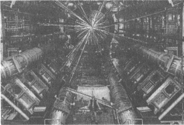
ŞEKİL 34 ATLAS'ta bir olayın dedektör katmanlarının arasından geçen enlemesine parçacık fışkırmasını gösteren simülasyonu. (Oradaki insan ölçeğin anlaşılmasına yardımcı oluyor ama insanlar dedektör bölgesindeyken çarpışmalar olmaz.) Farklı toroid mıknatıslar kolayca görülüyor (CERN ve ATLAS'ın izniyle).
