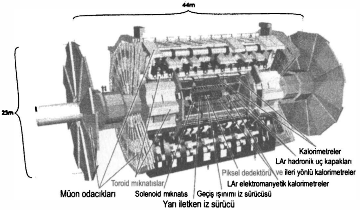
ŞEKİL 39 İç katmanları ve uç kapaklarını ayrılmış durumda gösteren ATLAS'ın bilgisayar görüntüsü (CERN ve ATLAS'ın izniyle).
