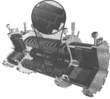
ŞEKİL 37 ATLAS'ın elektromanyetik kalorimetresinin akordeon şeklindeki yapısı.
