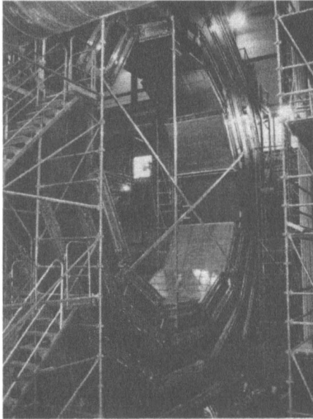
ŞEKİL 38 CMS'nin müon dedektörüyle geçmeli olan manyetik dönüş bobini, yapım halinde.
