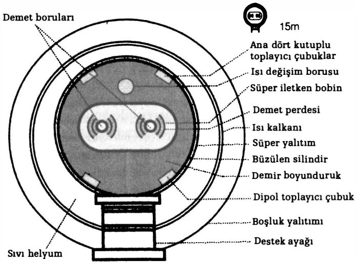
ŞEKİL 26 Bir kriyodipol mıknatısın şeması. Protonlar LHC çemberinde böyle 1232 adet süper iletken mıknatısın manyetik alanıyla turlarlar.
