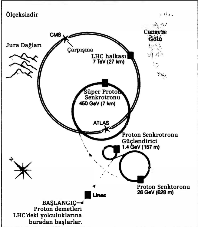
ŞEKİL 25 LHC'de hızlandırılan bir protonun izlediği yol.
