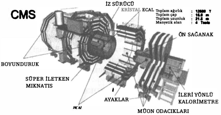
ŞEKİL 33 Dedektör parçalarının görülmesine olanak veren, CMS'nin parçalanmış bilgisayar görüntüsü. (CERN ve CMS'nin izniyle)
