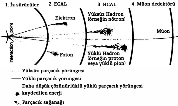
ŞEKİL 42 Standart Model parçacıklarının dedektörlerde nasıl ayırt edildiğinin bir özeti. Yüksüz parçacıklar iz sürücülerde görülmez. Hem yüklü hem de yüksüz hadronlar ECAL'de küçük birikimler bırakabilirlerse de enerjilerinin çoğunu HCAL'de depolarlar. Müonlar dış dedektörden geçer.
