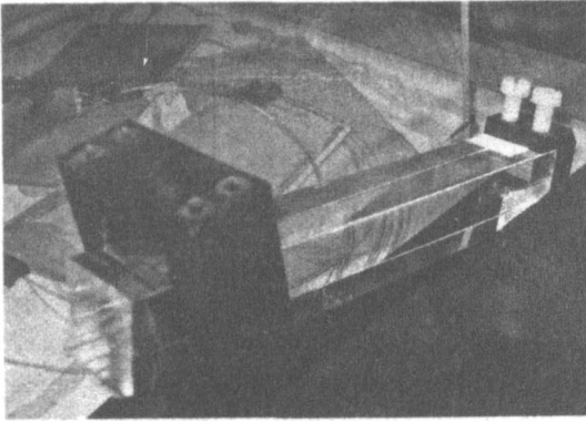
ŞEKİL 36 CMS'nin elektromanyetik kalorimetresinde kullanılan kurşun tungstat kristalinin fotoğrafı.
