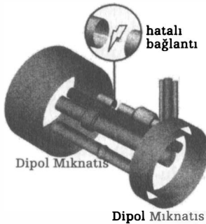
ŞEKİL 27 Farklı mıknatısları birleştiren toplayıcı çubuk. 2008'deki şanssız olaydan bu çubuklardan birindeki bir hatalı lehim sorumluydu.
