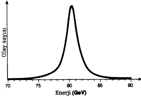
ŞEKİL 45 Bozunmuş parçacıkların ölçümleri gerçek kütlelerini merkeze alır ama kütleler yaşam sürelerine bağlı olarak bir dağılım gösterir. Şekil bunu W ayar bozonu için gösteriyor.
