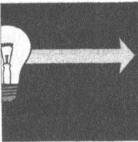
ŞEKİL 5 Geometrik optik ve dalga kuramı, ışığın modern kavrayışımızın öncüleri olup uygun koşullar altında hâlâ uygulanır.
