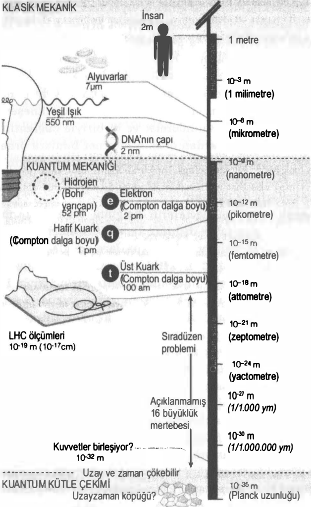
ŞEKİL 13 Küçük ölçeklere ve onları tanımlamakta kullanılan uzunluk ölçülerine bir gezinti.
