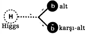
ŞEKİL 53 hafif bir Higgs bozonu esas olarak alt kuarklara bozunacaktır.
