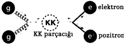
ŞEKİL 69 Randall-Sundrum modellerinde dedektörün içinde bir KK gravitonu üretilebilir ve elektronla pozitron gibi görülebilir parçacıklara bozunabilir.
