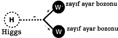
ŞEKİL 52 Çok ağır bir Higgs bozonu W ayar bozonlarına bozunabilir.
