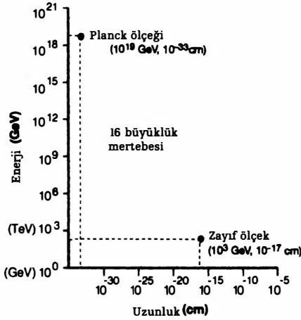
ŞEKİL 54 Parçacık fiziğindeki sıradüzen problemi: Zayıf enerji ölçeği kütleçekimle ilgili olan Planck ölçeğinden 16 büyüklük mertebesi daha küçüktür. Planck uzunluk ölçeği de LHC’de erişilebilen uzunluklardan aynı oranda küçüktür.
