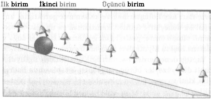
ŞEKİL 7 Geçiş i bildiren çanlar yardımıyla Galileo bir topun eğik düzlemde yuvarlanma hızını ölçtü.
