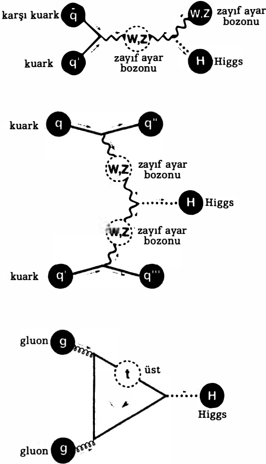
ŞEKİL 51 Higgs üretiminin üç kipi: sırayla (yukarıdan aşağıya, Higgs-strahlung, WZ füzyonu ve gg füzyonu.
