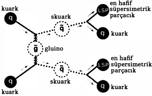
ŞEKİL 60 LHC’de, her ikisi de kuarklara ve LSP’lere bozunan ve kayıp enerji imzası veren iki skuark birlikte üretilebilir.
