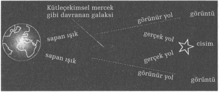
ŞEKİL 75 Büyük kütleli bir cismin yanından geçen ışık bükülebilir ve gözlemcinin baktığı yerden özgün cismin çoklu görüntüsü yaratılmış gibi görünür.
