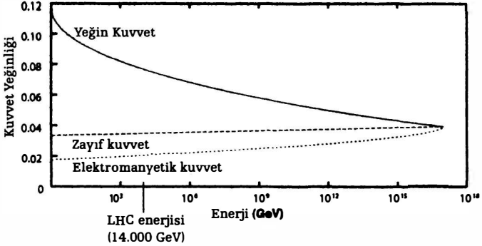
ŞEKİL 19 Yüksek enerjilerde kütleçekim dışında bilinen üç kuvvet aynı yeğinliğe sahip olabilir, dolayısıyla tek bir kuvvet altında birleşebilir.
