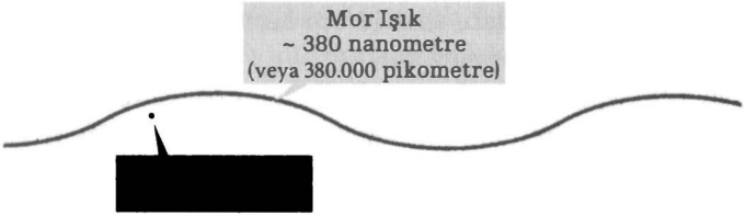
ŞEKİL 14 Bir atom, görülür ışığın en kısa dalga boyuyla bile karşılaştırıldığında sadece bir noktadır.
