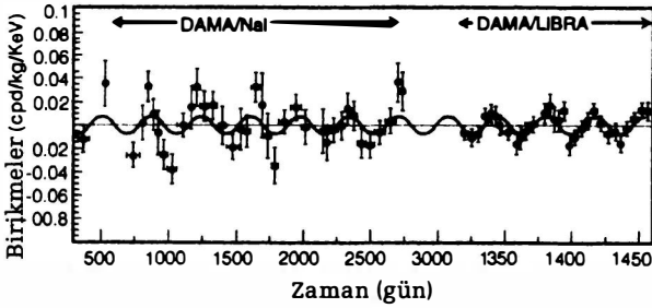
ŞEKİL 79 DAMA deneyinin, sinyalin zamana göre modülasyonunu gösteren verileri.
