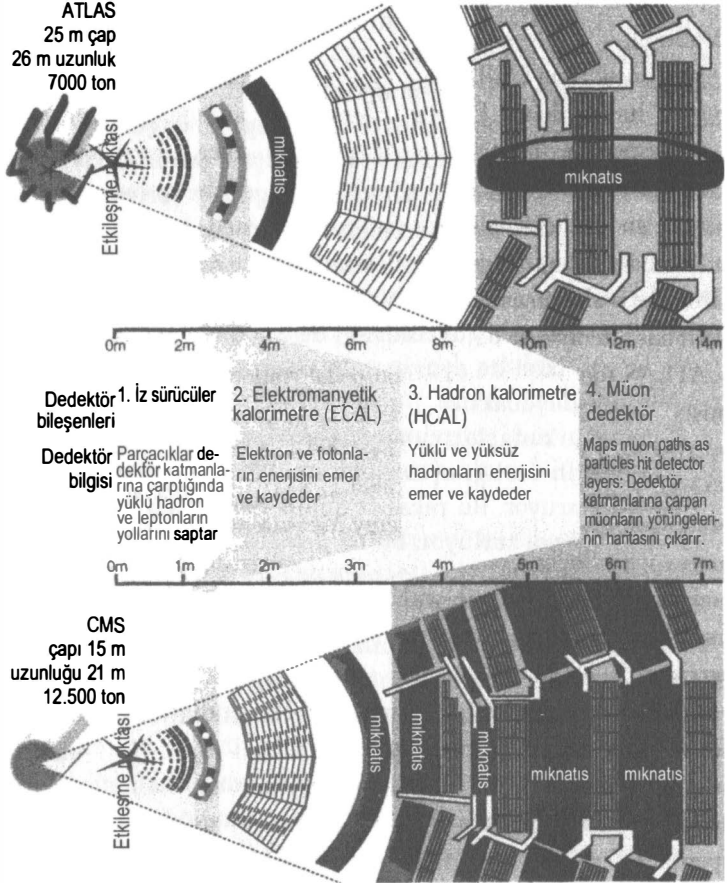
ŞEKİL 32 ATLAS ve CMS dedektörlerinin kesitleri. Genel boyutların yeniden ölçeklendirildiğine dikkat ediniz.
