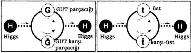
ŞEKİL 55 Higgs bozonu kütlesine ağır bir parçacıktan –örneğin GUT kütle ölçekleriyle– ve bunun karşı-parçacığından gelen ( solda ) ve sanal bir üst kuark ve bunun karşı-parçacığından ( sağda ) gelen kuantum katkıları.
