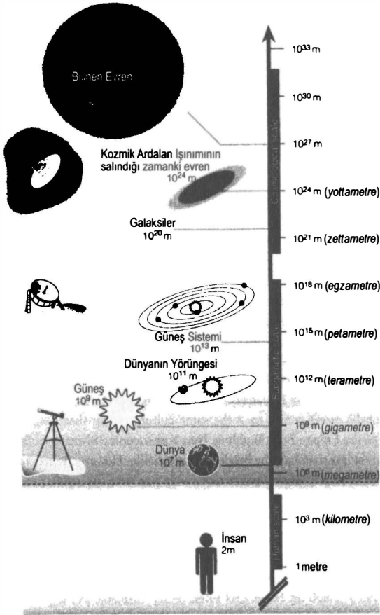
ŞEKİL 70 Büyük ölçeklerde bir tur ve bunları tanımlamakta kullanılan uzunluk ölçüleri.
