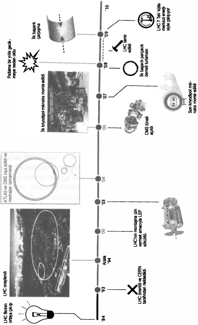
ŞEKİL 28 LHC tarihinin ana hatlarının özeti.
