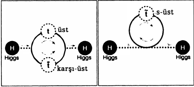
ŞEKİL 58 Süpersimetrik bir modelde sanal süpersimetrik parçacıkların Higgs bozonunun kütlesine olan katkıları Standart Model parçacıkların katkılarını yok eder. Örneğin yukarıdaki iki diyagramda görülen katkıların toplamı sıfırdır.
