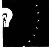
ŞEKİL 5 Geometrik optik ve dalga kuramı, ışığın modern kavrayışımızın öncüleri olup uygun koşullar altında hâlâ uygulanır.
