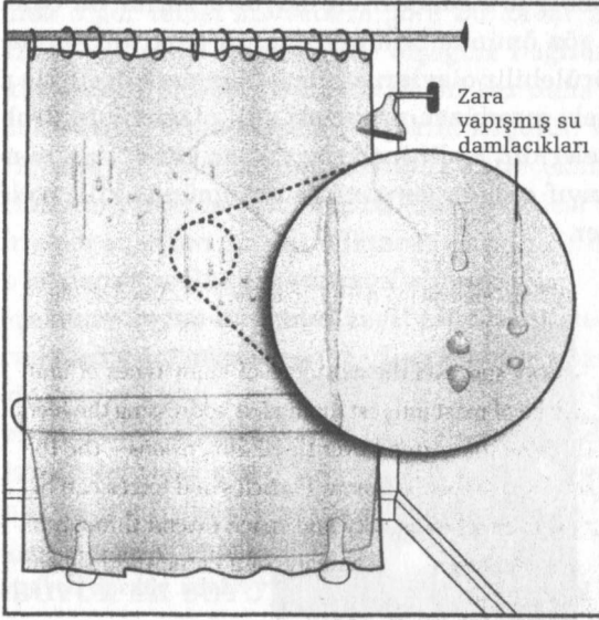
ŞEKİL 62 Bir zarın yakaladığı parçacık ve kuvvetler zar yüzeyi boyunca hareket edebilir ama oradan ayrılamazlar, tıpkı duş perdesi üzerinde hareket edebilen ama oradan ayrılamayan su damlacıkları gibi.
