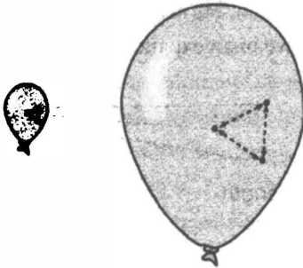
ŞEKİL 72 “Balonevren”, balon (evren) genişlerken bütün noktaların birbirinden nasıl uzaklaştığını gösteriyor.
