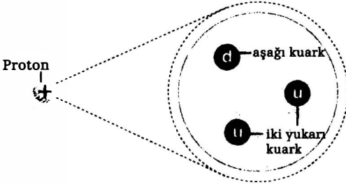
ŞEKİL 16 Protonun yükü üç değerlik kuarkı, iki yukarı ve bir aşağı kuark tarafından taşınır.
