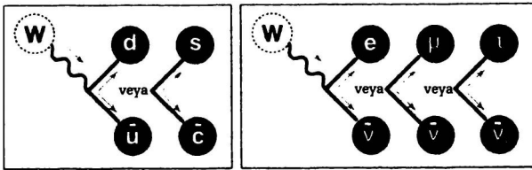
ŞEKİL 44 W bozonu yüklü bir lepton ve onunla ilgili nötrinoya veya bir yukarı ve bir aşağı kuarka ya da bir tılsımlı ve bir acayip kuarka bozunabilir. Gerçekte bu fiziksel parçacıklar farklı türde kuark ve nötrinoların bir üstdüşümüdür. Bu durum W 'nin zaman zaman eşanlı olarak farklı kuşaktan parçacıklara bozunumuna olanak sağlar.
