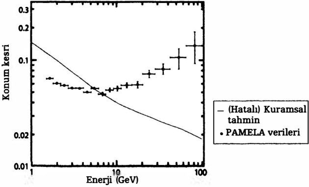
ŞEKİL 80 PAMELA deneyinde deneysel verilerin (noktalar) kuramsal hesaplarla (noktalı eğri) uyuşmadığını gösteren grafik.
