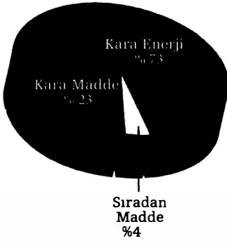
ŞEKİL 74 Evrenin yapısında bulunan görülür madde, kara madde ve kara enerjinin göreceli miktarlarını gösteren grafik.
