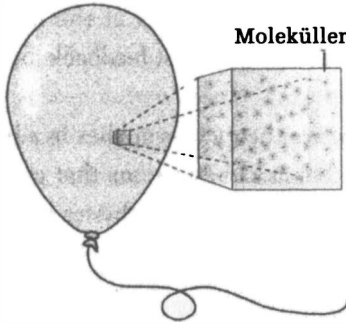
ŞEKİL 4 Basınç ve sıcaklık, çok daha temel düzeyde, tek tek moleküllerin fiziksel özellikleri cinsinden anlaşılabilir.
