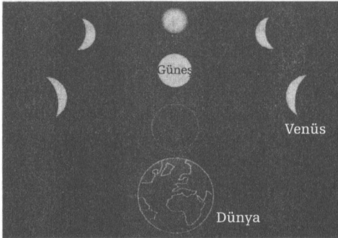
ŞEKİL 9 Galileo'nun Venüs'ün evreleri konusundaki gözlemleri, onun da güneşin etrafında döndüğünü göstererek Ptolemaios sisteminin geçerli olmadığını gösterdi.
