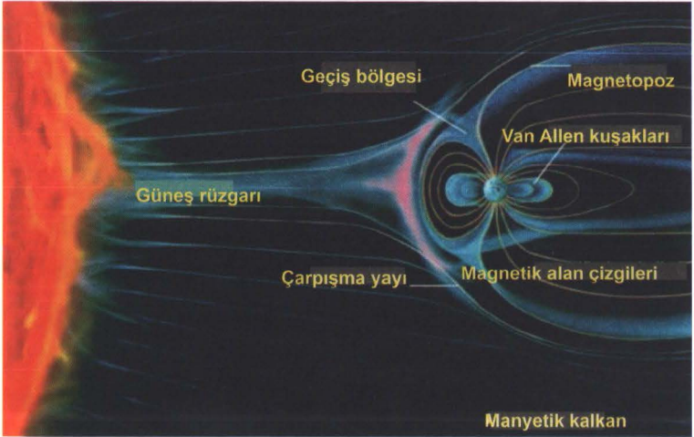
Şekil 9: Bundan yaklaşık 4,8 milyar yıl önce, Dünya'yı yıkıcı Güneş ışınlarından koruyan "Allen Kuşakları", manyetik kuşaklar ortaya çıktı ( www.tpscernbilim.blogspot.com/201803van-allen-kusagndan-gecilemezmi.html ).
