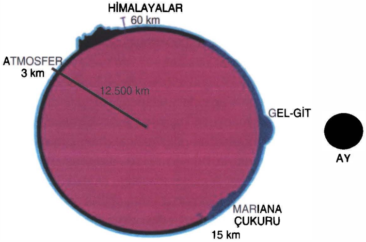
Şekil 8: İki gezegenin çarpışması ile ortaya çıkan Ay, kütle çekiminden dolayı Dünya'da bir elektromotor gücünün, bu da elektrik alanının, o da manyetik alanların ortaya çıkmasını sağlar.
