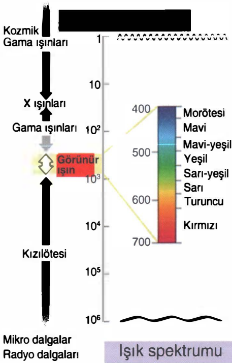
Şekil 15: Güneş'ten çıkıp, Allen Kuşakları'na ve ozon tabakasına ulaşan Güneş ışınlarının profili ve bizim algılama sınırlarımızın içine giren kesimi: Görünür ışın dalgaları.
