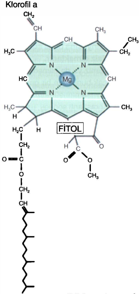
Şekil 19: Klorofilin yapısı.
