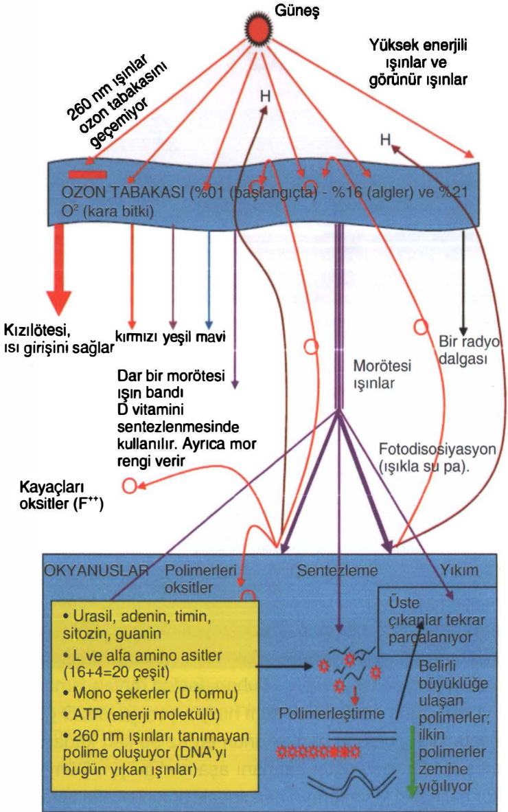
Şekil 13: İlk ve ilkin ozon tabakasının oluşumu ve fotodisosiyeasyon olayının gerçekleşmesi.
