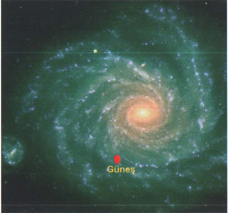
Şekil 4: Samanyolu Galaksisi ve Güneş'in konumu (İnternette).
