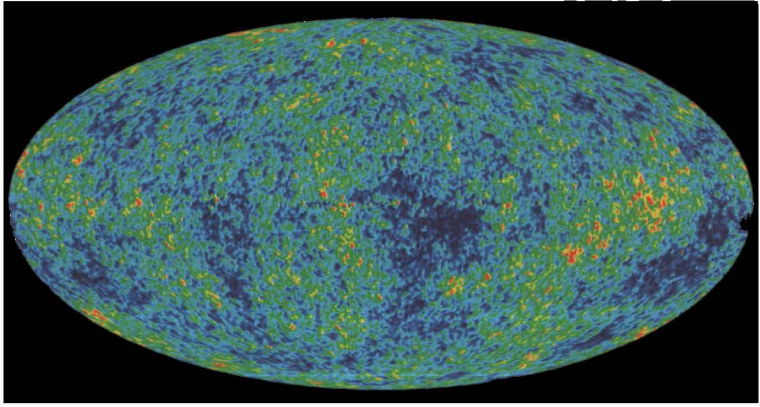
Şekil 2: Bugün Evren'in kozmik arka plan mikrodalga dağılımına baktığımızda şöyle bir yapı olduğunu söyleyebiliriz.
