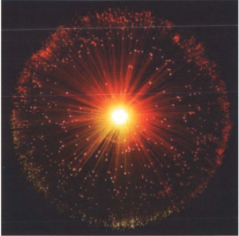
Şekil 1: Sürekli Evren'den 13,7 milyar yıl önce patlama ile bugünkü Evren oluşumu başladı (İnternetten).
