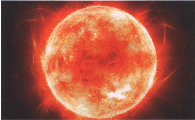
Şekil 5: Bundan 5,5 milyar yıl önce Samanyolu'nun merkezine yakın, orta boy bir yıldız oluşuyor. Bunun adı Güneş'tir (İnternette).
