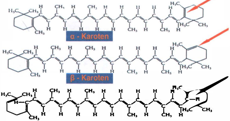
Şekil 174: Renkleri veren pigmentlerde bir bağı değişmesi ya da küçük bir molekülün bağlanması ya da yer değiştirmesi rengin değişimine neden olur.
