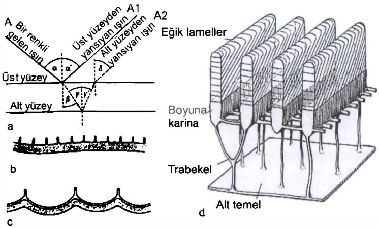
Şekil 167: Canlıların bir kısmında tabaka tabaka konumlanmış keratin katmanlarının Güneş ışığının bazı dalga boylarını yansıtıp, bazı kısımlarını absorbe etmesi ile yansıyan ışığın denk geldiği renk görülür.
