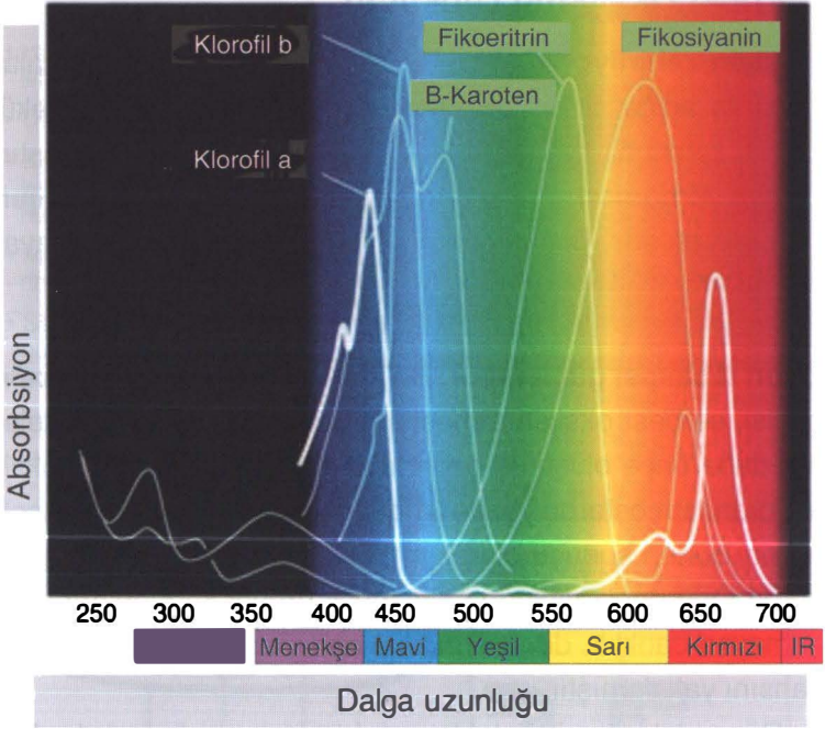
Şekil 20: Güneş ışığının klorofil tarafından absorbe edilen ve soğurulan dalga boyları. Dikkat edilirse yeşil renk hiç soğurulmadığı ve yansıtıldığı için bitkiler yeşil renkli görünür.
