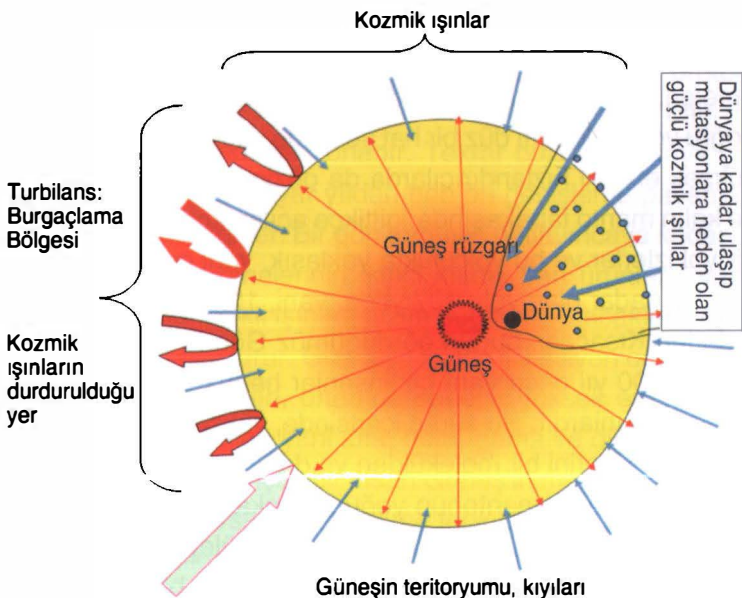
Şekil 7: Güneş'ten çıkan ışınların kozmikten gelen ışınlar ile çarpışıp, kendi gezegenlerini koruması.
