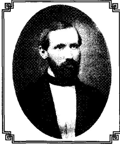
Bernhard Riemann (1826-1866)
