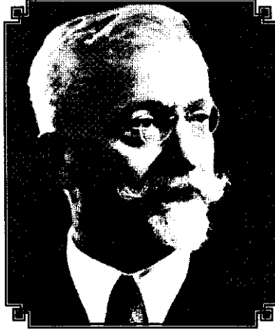
Elie Cartan (1869-1951)
