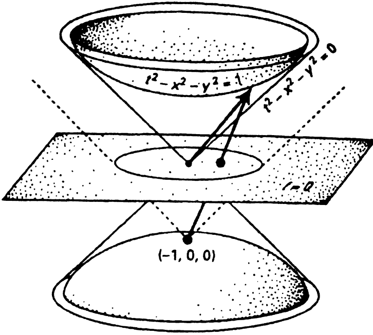
Şekil 1.21. Lobachevski uzayının bir hiperboloit şube halinde Minkowski uzay-zamanı içine yerleştirilmesi. Stereografik izdüşüm bu hiperboloiti, t=0 düzlemi üzerinde çizili sınırlandırılmış olan Poincaré diskine eşle-mektedir.
