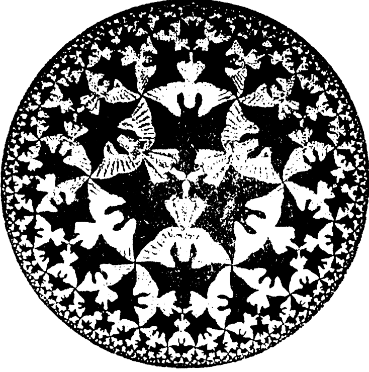
 ekil 1.17. M. C. Escher'in " ember Sınır 4" adlı eseri (Lobachevski uzayının tipik bir temsili).
