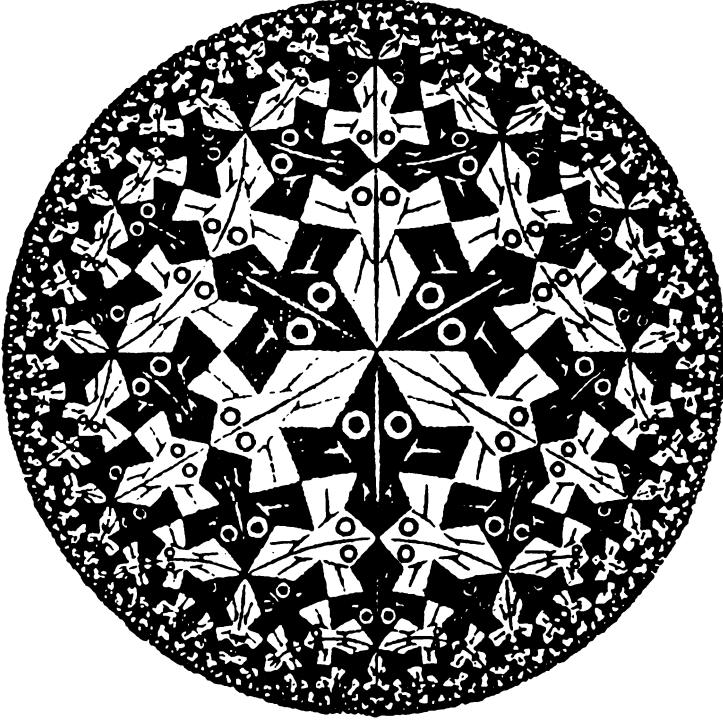
Şekil 1.19. M. C. Escher'in "Çember Sınır 1" adlı eseri.
