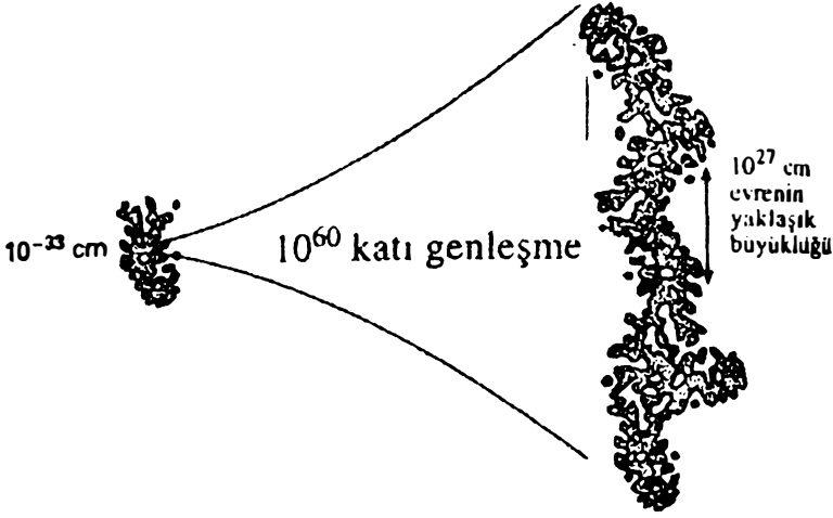
Şekil 1.27. Evren'in ilk dönemlerinde rastlanan "ne idüğü belirsiz" düzensizliklerin genişlererek büyümeleri problemi.
