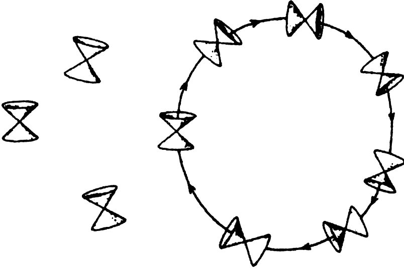
Şekil 3.13. Uzay-zaman içinde ışık konilerinde yeterince şiddetli bir bükülmenin meydana gelmesi durumunda, zaman yerine geçen kapalı akışların oluşması mümkündür.
