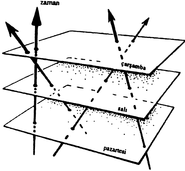
Şekil 1.6. Galilei uzay-zamanı: düzgün biçimli hareket halinde olan parçacıklar düzgün doğrularla gösterilmektedir.
