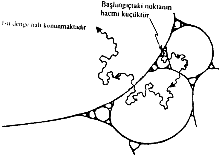
Şekil 1.25. Termodinamiğin İkinci Yasası ışığında: zaman ilerledikçe, faz uzayında seçilen nokta gitgide daha büyük hacimli bölmelerin içine gitmektedir. Buna bağlı olarak da entropi sürekli artmaktadır.
