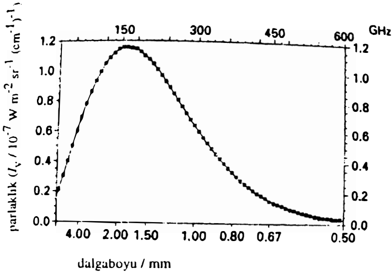
Şekil 1.22. Evrensel Mikrodalga Arkaalan Işıması tayfını saptamak üzere yapılan COBE ölçümleri ile Büyük Patlama'dan arta kalan ışımanın beklenen "ısı" karakteri (kesiksiz çizgi) arasında yüksek bir isabet vardır.
