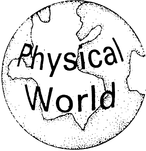
Şekil 1.1 — Fiziksel Dünya
