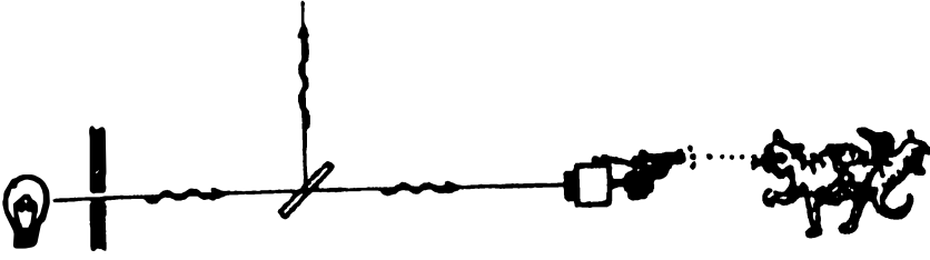
Şekil 2.7. Schrödinger'in kedisi. Kuantum hali, bir fotonun yansıtılan ve iletilen bileşenlerinin lineer bir tarzda üst üste binmesinden oluşmaktadır. İletilen bileşen, kediyi öldüren bir düzeneği harekete geçirmektedir. Böylelikle U-gelişimine göre kedi, ölümle dirimin üst üste bindiği bir halde varolmayı sürdürmektedir.
