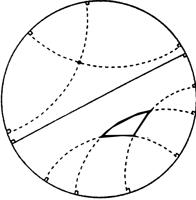
Şekil 1.20. "Circle Sınır 1'de betimlenen Lobachevski (hiperbolik) uzayı geometrisinin bazı özellikleri.
