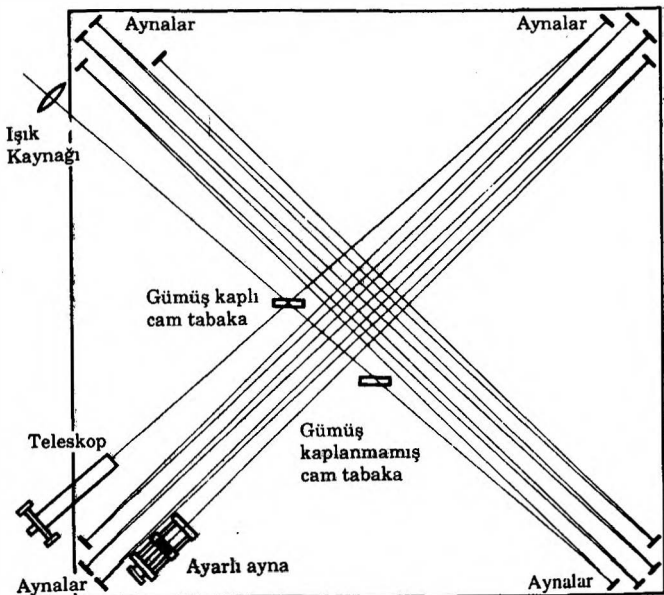
Şekil 25. Düzenegın son durumunu gösteren diyagram. Michelson ile Morley'in 1887 yılında yayımlanan çizimi, üçüncü seri, Cilt 34..
