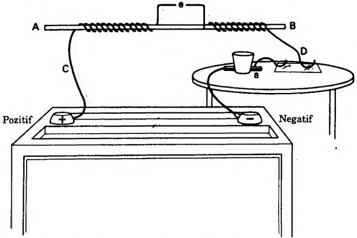
Şekil 34. Voltaik elektrik deşarjını kanıtlamak için geliştirilen aygıt.
