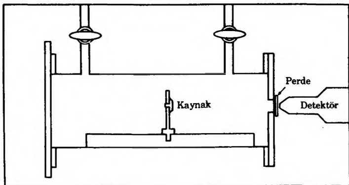
Şekil 21. Deneyel düzenleme.
