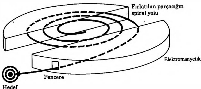
Şekil 22. Hızlandırıcıda ışının izlediği yol.
