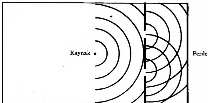
Şekil 2. Dalgaların parazit kalıbı. Tek tek elektronların tüm fiziksel özelliklerinin tam olarak ölçülmesinden önce, katı bir perde üzerindeki yarıklardan salınan elektron demetleri dalga gibi davranıyor.
