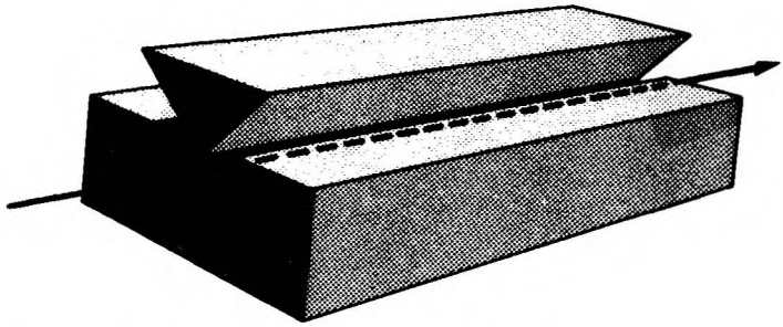
Şekil 38. Stern-Gerlach aygıtı içindeki elektro nuktasının kutup parçaları.
