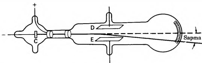
Şekil 29. Deneyel düzenleme. C Katot ışınlarının kaynağıdır.
