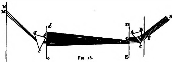
Şekil 30. "Kırınım"ı farklı olan ışınların ayrışması. Newton, Opticks , (1721 basımı), birinci kitap, 1. bölüm, tablo IV, fig. 18 s, beyaz ışığın kaynağını gösteriyor. Kırınımını farklı olan ışınlar ABC prizmasında ayrıştırıyor. DE ve de perdeleri, giderek daha net renkler elde etmeye yarıyor.
