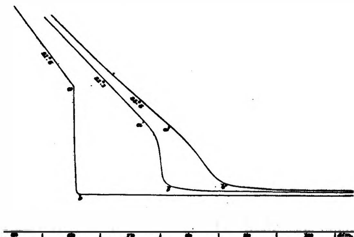
Şekil 16. Hacim ile basınç arasındaki ilişkilerin Boyle Yasasına uymadığı anlar. Eğrinin basınç eksenine paralel olduğu "kritik nokta"ya yaklaştıkça gaz sıvılaşır. T. Andrews, Bakerian Lecture, "Maddenin Gaz Hali", Philosophical Transactions of the Royal Society Cilt.166 (1876), Sayfa 443.
