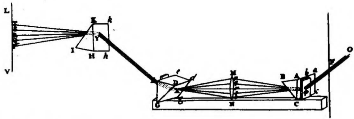
Şekil 32. Beyaz ışığın tayfa ayrışması, yeniden birleşmesi ve yeniden ayrışması. Newton, Opticks (1721 basımı), 1. Kitap II. bölüm, tablo IV şekil 16. ABC prizmasının yeniden kırıldığı ışınlar MN merceğiyle tekrar birleştiriliyor, sonra KIH prizmasıyla tekrar ayrıştırılıyor.
