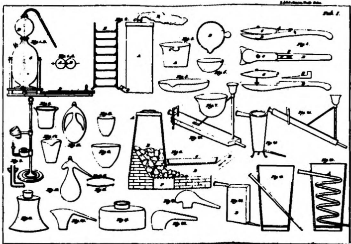
Şekil 35. Berzelius'un geliştirdiği düzeneklerden örnekler. "Kimya üzerine Denemeler"ın özgün İsveççe baskısından alınmıştır. Cilt III, Tablo 1.
