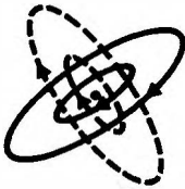
Nicelenmiş yörüngesel düzlemler
