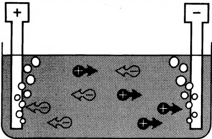
Şekil 28. İyonların Göçü.
