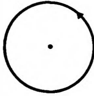
Nicelenmiş açısal nomentum
