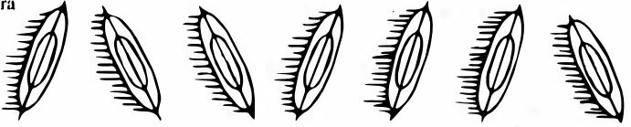
Şekil 39. Atomların yöneliminde manyetik alanın değiştirilmesinin etkisi
