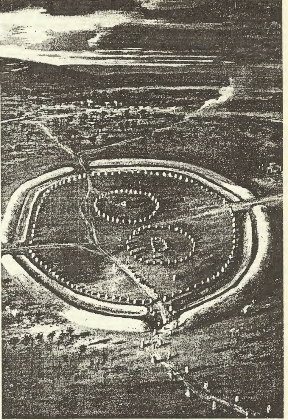
Avebury megalitleri.
