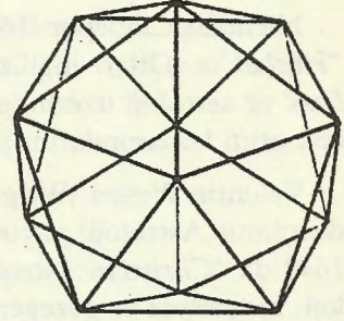
İkozahedron
