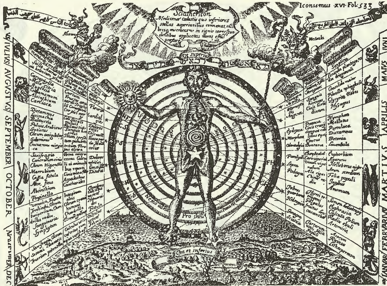
Kircher'e göre insan bedeninin astrolojik ve hermetik karşılıkları.
