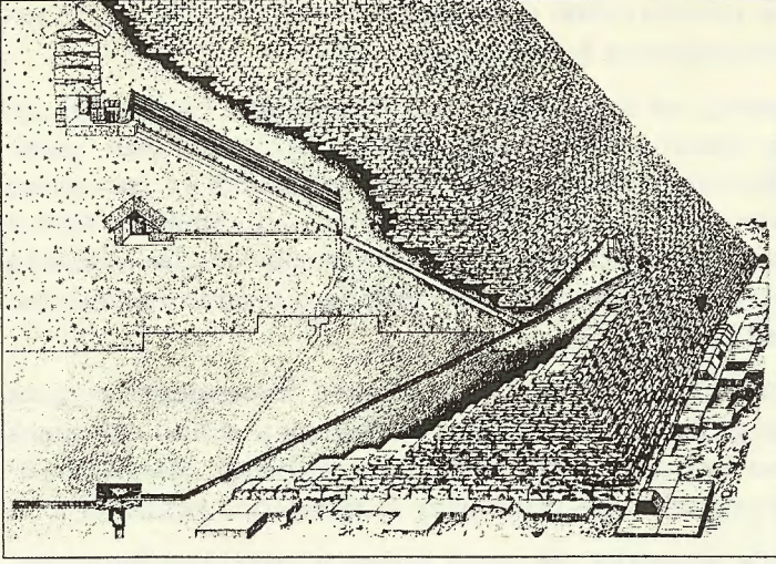
Büyük Piramit'in, geçitlerini Kral Odası'nı gösteren kesit.
