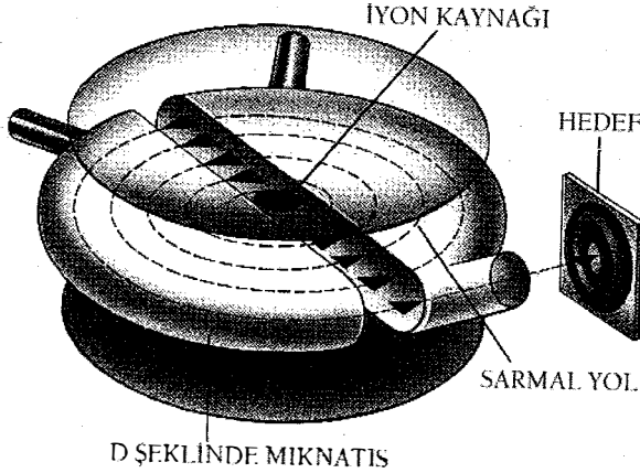
Siklotronda iyonlar makinenin merkezinde üretilir. Hedefe doğru hızlanırlarken manyetik bir alan sarmal bir yol izlemelerini sağlar.
