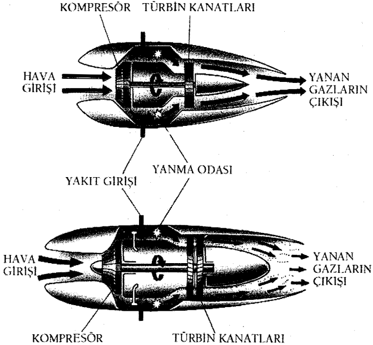
Whittle'in orijinal jet motorunun (yukarıda) öndeki kompresörü çalıştıran tek bir türbini vardı; daha sonraki motorlarda (aşağıda) iki ya da daha fazla türbin kanatları yer aldı.
