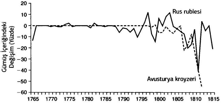
Şekil 11.1. Para biriminin içerdiği gümüş miktarındaki değişimler, 1765-1815:
