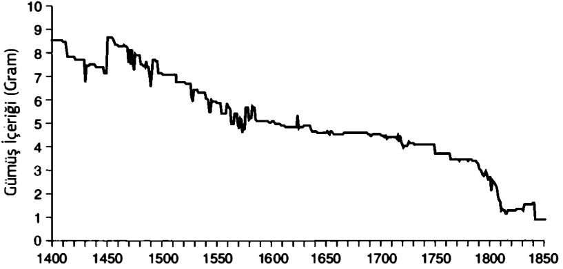
Şekil 11.2. Fiat (kağıt) paraya doğru gidiş, Avrupa, 1400-1850:
