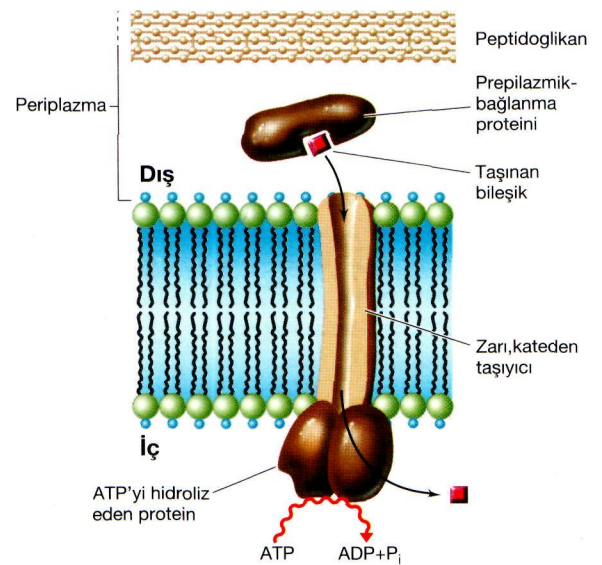
• Şekil 4.26 ATP-Bağlayan Kaset taşıyıcının (ABC-tipi) mekanizması. Periplazmik bağlanma proteini substrata karşı yüksek ilgi gösterir, zarı kateden protein taşıma kanalı olarak iş görür, sitoplazmik ATP-hidroliz eden protein ise taşıma olayı için enerji sağlar. Escherichia coli 'deki maltoz taşıyan sistem ABC sistemine bir örnektir. Gram-negatif duvar yapısı ve periplazma konusu Kısım 4.9'da anlatılmaktadır.
