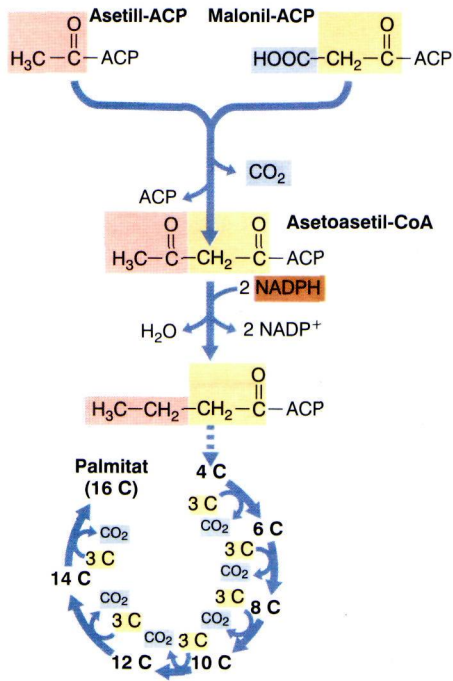
♦ Şekil 5.29 Yağ asitlerinin biyosentezi. Palmitat'ın (C 16 yağ asidi) biyosentezi (Şekil 3.7). Asetil-ACP ile malonil-ACP'nin kondensasyonu sonucunda asetoasetil-CoA oluşur. Birbiri ardına eklenen her bir asetil birimi malonil-ACP'den gelmektedir.
