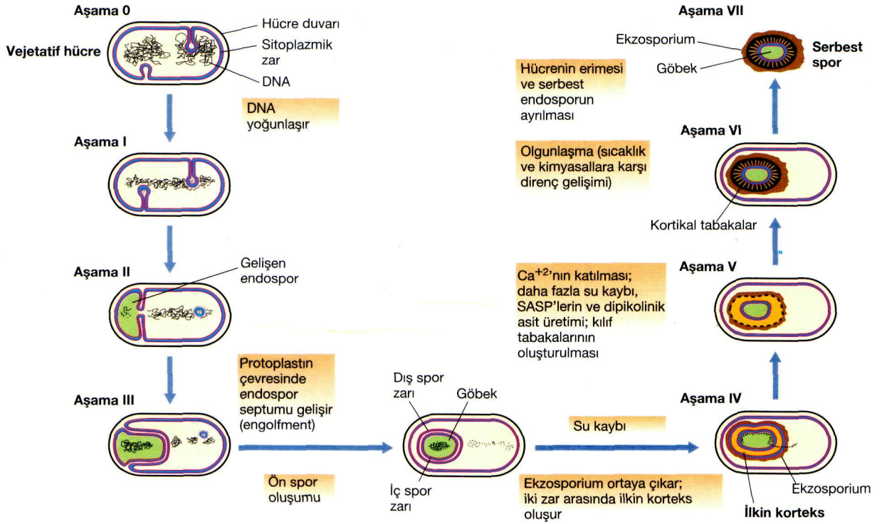
● Şekil 4.51 Endospor oluşum aşamaları. Listelenen aşamalar (0-VII) hem genetik çalışmalar, hem de mikroskopik analizlerle ortaya çıkarılmıştır.
