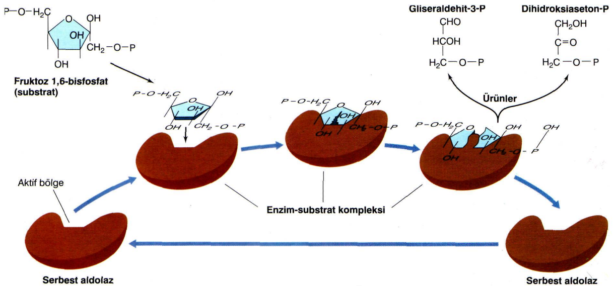
• Şekil 5.6 Fruktoz bisfosfat aldolaz enziminin katalitik döngüsü. Bu enzim glikoliz sırasında fruktoz 1,6-bisfosfat → gliseraldehit 3-fosfat + dihidroksiaseton fosfat tepkimesini katalizler (Bkz. Şekil 5.14). Enzim-substrat kompleksinin oluşumu sırasında, fruktoz 1,6-bisfosfat molekülünün bağlanmasını takiben enzimin konformasyonu değişir ve substratın belirli bağları üzerine baskı uygulanır. Bu baskı substratın iki ürün oluşturmak üzere kırılmasına yol açar.
