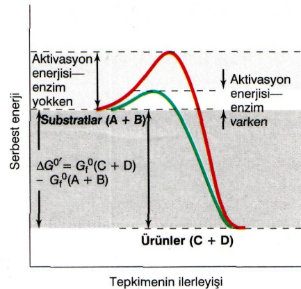
• Şekil 5.5 Hipotetik bir ekzergonik tepkimenin ilerleyişi: A + B \rightarrow C + D , ve aktivasyon enerji kavramı. Enerji açığa çıkışı ile gerçekleşen kimyasal tepkimeler bile kendiliğinden cereyan edemeyebilir. Aktivasyon sağlandıktan sonra, tepkime kendiliğinden ilerler. Enzim gibi katalizörler, tepkime için gerekli olan aktivasyon enerjisini düşürürler.
