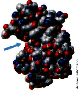
● Şekil 5.7 Lizozim enziminin bilgisayarda oluşturulmuş uzay modeli. Substrat (peptidoglikan) bağlama bölgesi (aktif bölge), modelin sol tarafında okla gösterilen geniş girintidir.
