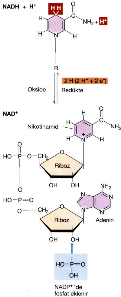
♦ Şekil 5.10 Oksidasyon-redüksiyon koenzimi olan nikotinamid adenin dinükleotit (NAD + )'nin yapısı. NADP + yapısında ok ile gösterilen kısımda bir fosfat grubu bulunur. Hem NAD + hem de NADP + gösterildiği gibi oksidasyon-redüksiyona uğrar, serbestçe difüze olur ve 2e - + 2H + taşırlar. Diyagramın üst kısmındaki "R", NAD + 'nin adenin dinükleotit kısmı olup, molekülün tamamı diyagramın alt kısmında gösterilmiştir.
