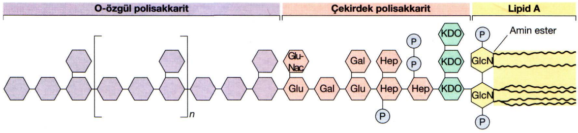
● Şekil 4.34 Gram-negatif Bacteria'daki lipopolisakkarit yapısı. Çeşitli gram-negatif Bacteria türlerindeki lipid A ve polisakkarit bileşenlerin kimyasal yapıları değişmekle birlikte, temel bileşenlerin sıralanışı genelde değişmeden kalır (lipid A-KDO-çekirdek-O-özgül). O-özgül polisakkarit türler arasında farklılık gösterir. KDO, ketodeoksioktonat; Hep, heptoz; Glu, glukoz; Gal, galaktoz. Amin ester lipid A'nın yağ asitleri arasındaki bağ, amin ester bağıdır. LPS'nin lipid A kısmı, endotoksin kompleksini oluşturur ve hayvanlarda toksik etki yapabilir (Kısım 21.12). Bu şekli Şekil 4.35 ve 4.36 ile karşılaştırdınız. Şekil 4.34 ve 4.35'deki LPS'nin farklı kısımlarında kullanılan renk kodlarına dikkat ediniz.
