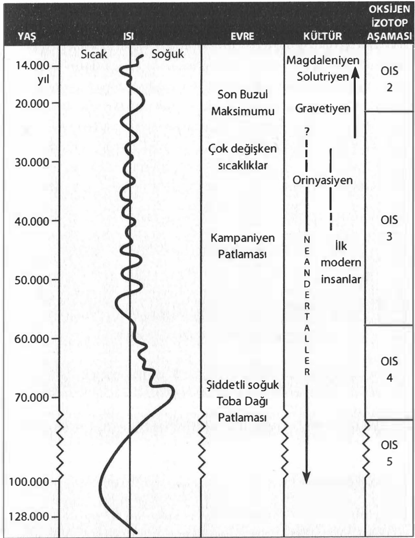
Şekil 3.3 Son Buzul Çağı'nın iklim değişikliğini Avrupa'daki önemli kültürel gelişimleriyle birlikte gösteren genel bir özet.
