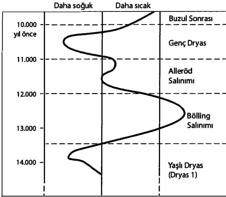
Şekil 12.2 Son Buzul iklim değişimi.
