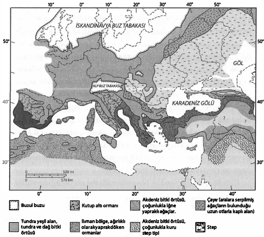
Şekil 8.1 Son Buzul Maksimumu'nda Avrupa
