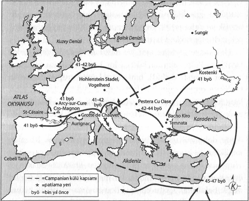
Şekil 6.3 Avrupa'nın modern insan yerleşimi, Kampaniyen patlamasından yayılan külün yaklaşık alanını da göstermektedir.
