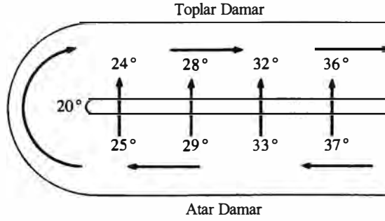
Şekil 15.2 Ters akıntı çoklu sistemi
