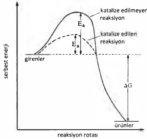
Şekil 3.3 Katalize edilmeyen reaksiyon, katalize edilen reaksiyona göre daha yüksek aktivasyon enerjisi, E_a gerektirir. \Delta G kimyasal reaksiyonda salınan enerji miktarını gösterir ve katalize edilen ve edilmeyen reaksiyonlarda aynıdır.
