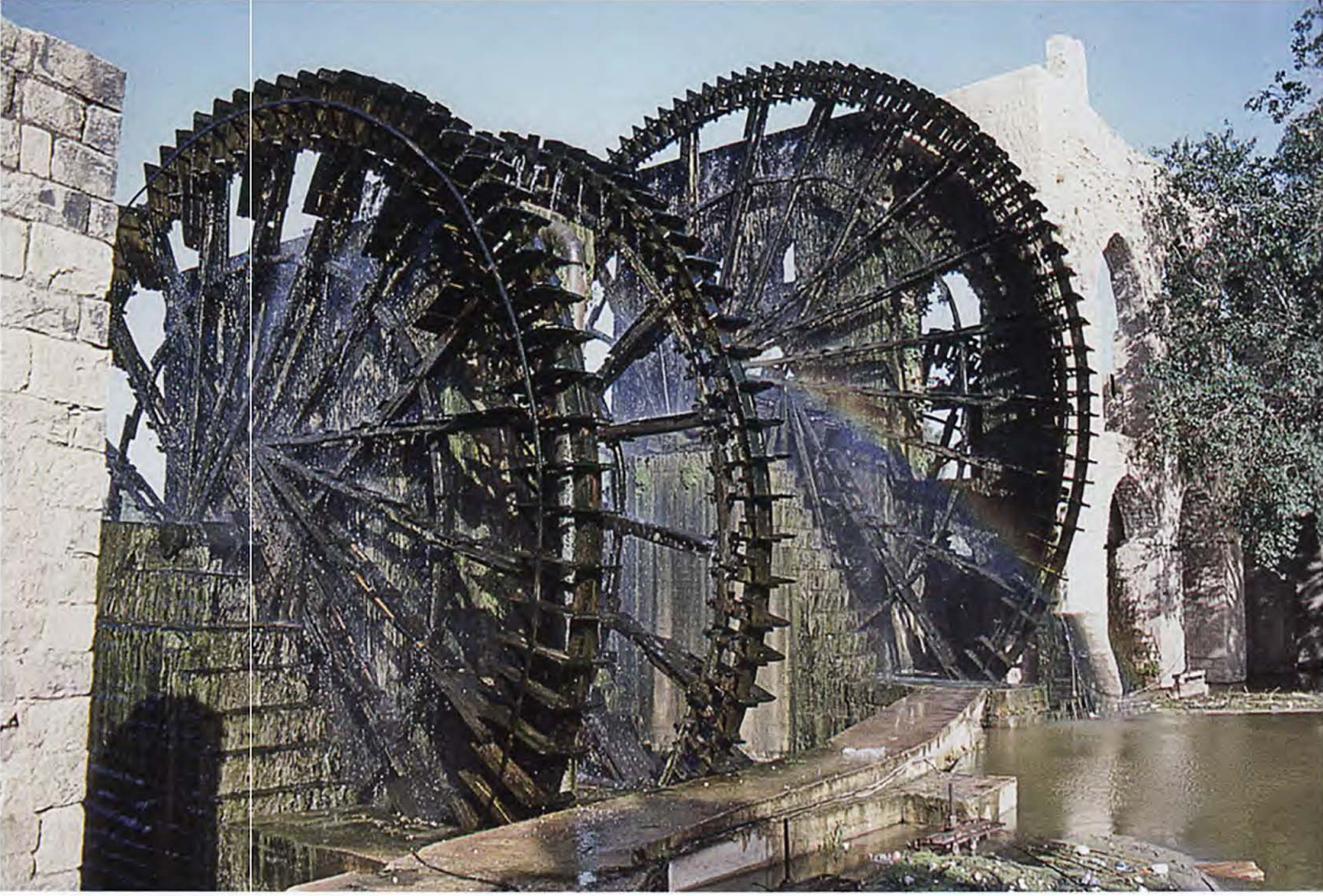
Suriye'nin Hama şehrinin kuzeyindeki dış mahallelerden birinde, Asi Nehri üzerinde, Ortaçağ'dan kalma dört adet değirmen çarkı (Yazarın çektiği fotoğraf).
