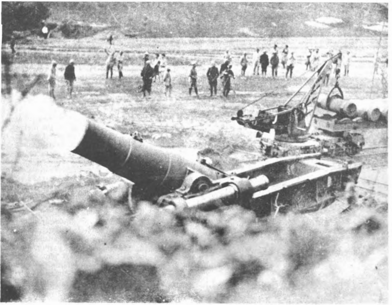
Fransızların bu savaşta ilk kez kullandıkları 270 mm'lik toplardan biri.
